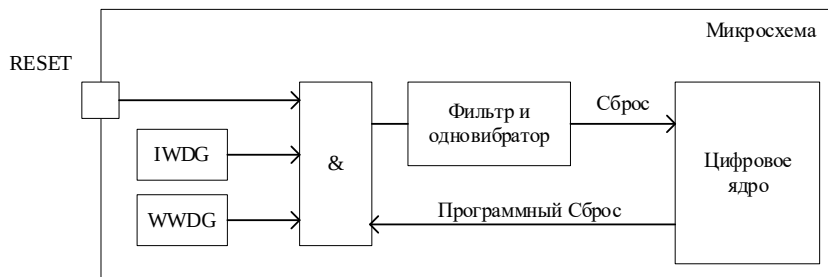
Рисунок 13 – Структурная блок-схема сброса
