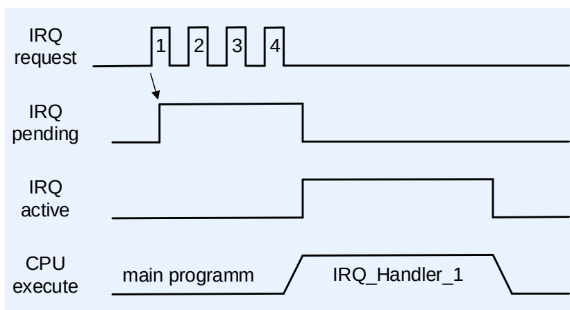
Рисунок 147 – Многократная установка снятие запроса IRQ request
