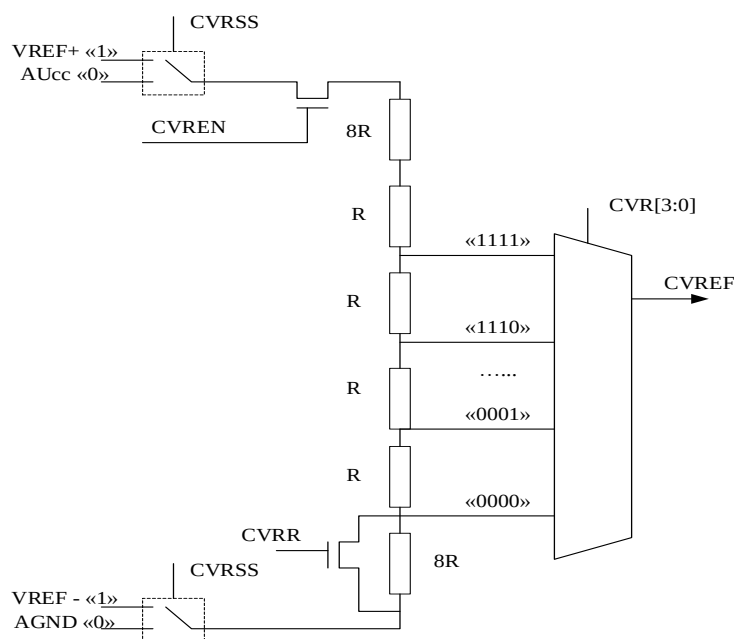
Рисунок 102 – Структура блока формирования CVREF
