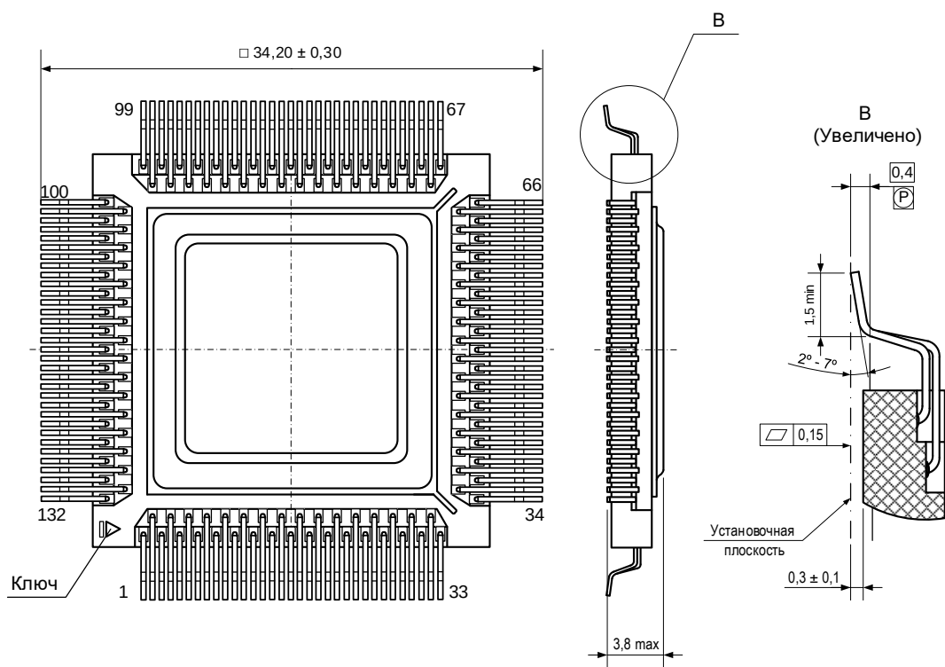
Рисунок 159 – Габаритный чертеж микросхемы в корпусе 4229.132-3 с формованными выводами
