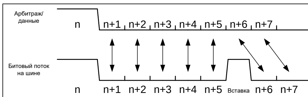
Рисунок 65 – Битстаффинг
