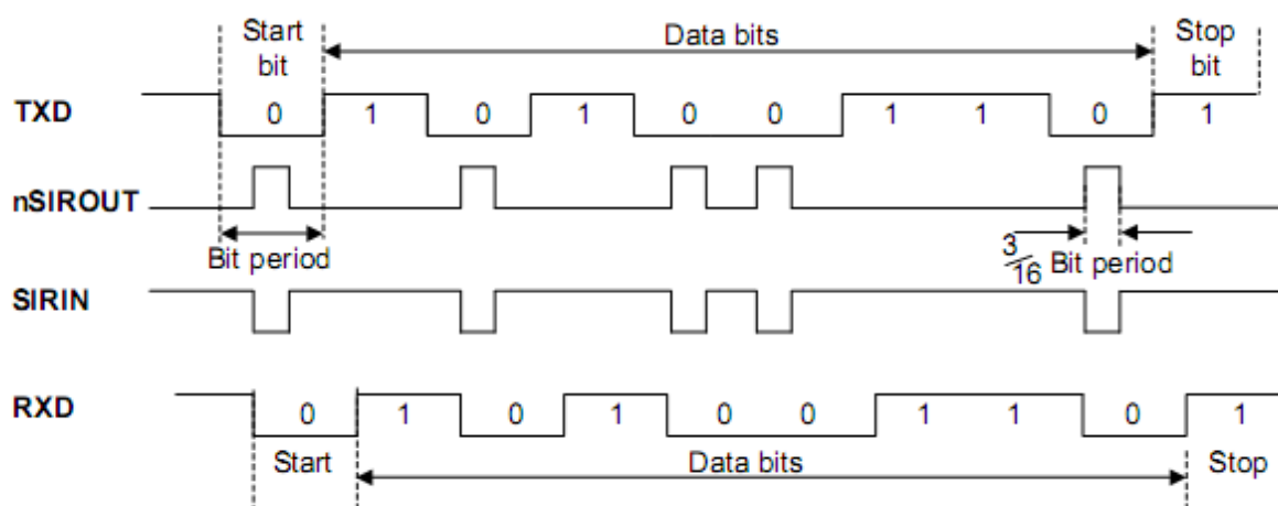
Рисунок 126 – Модуляция данных IrDA
