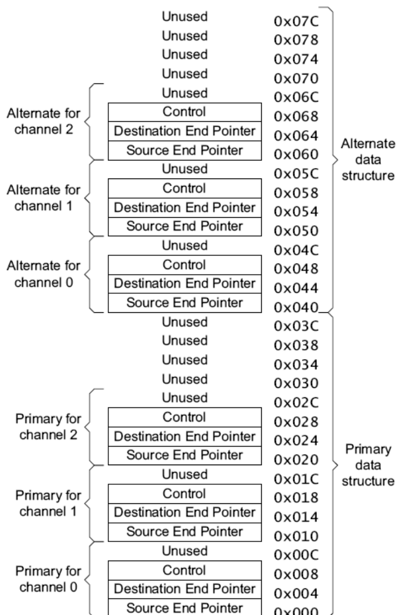
Рисунок 140 – Карта памяти для трех каналов DMA, включая альтернативную структуру
