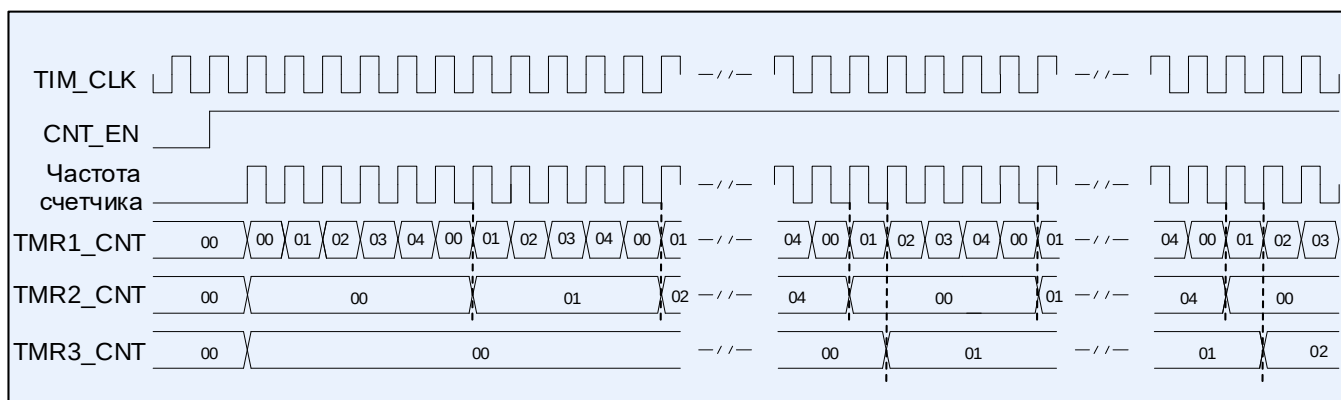
Рисунок 79 – Диаграммы работы трех таймеров в каскаде
