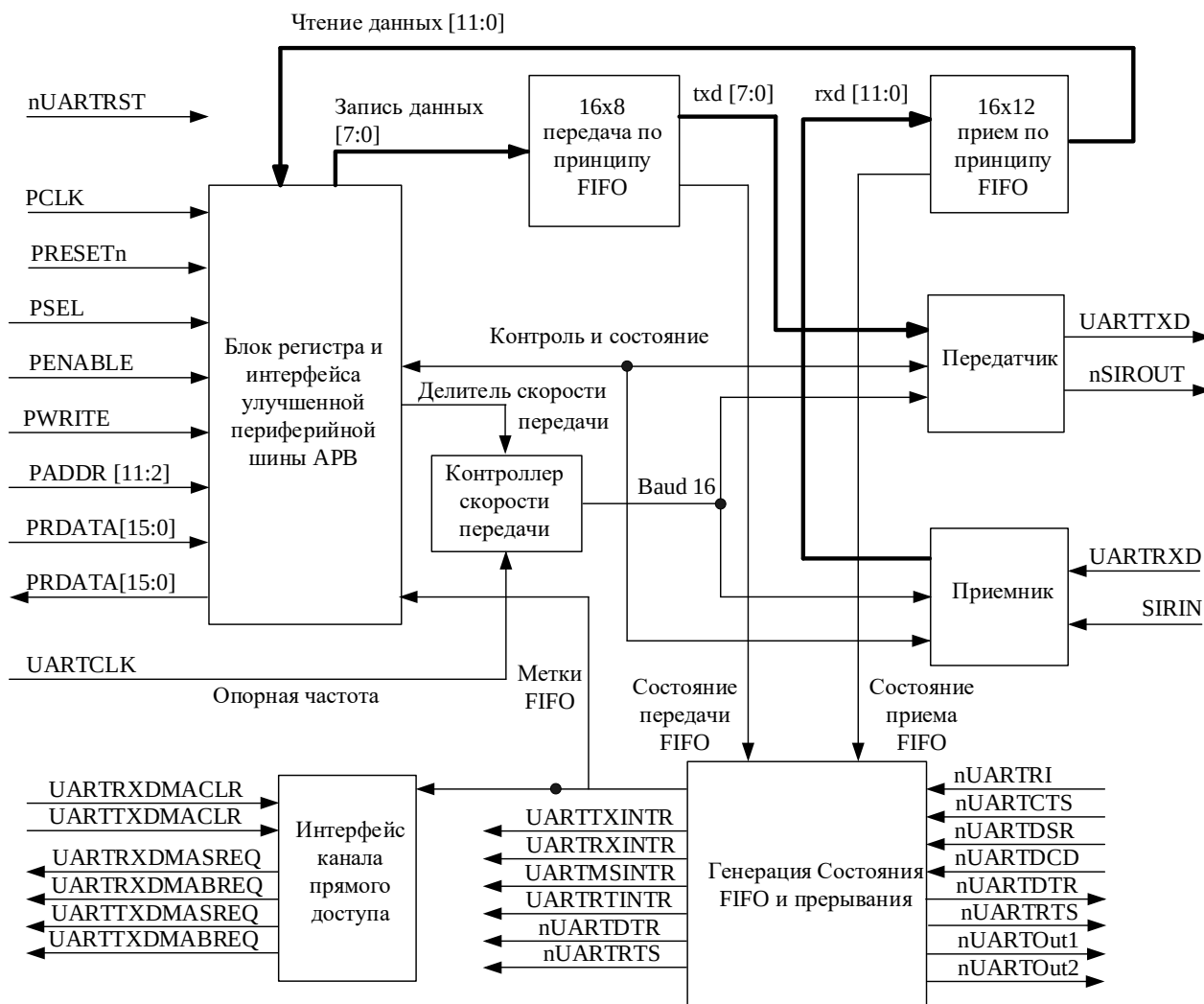
Рисунок 122 – Блок-схема универсального асинхронного приемопередатчика (UART)
