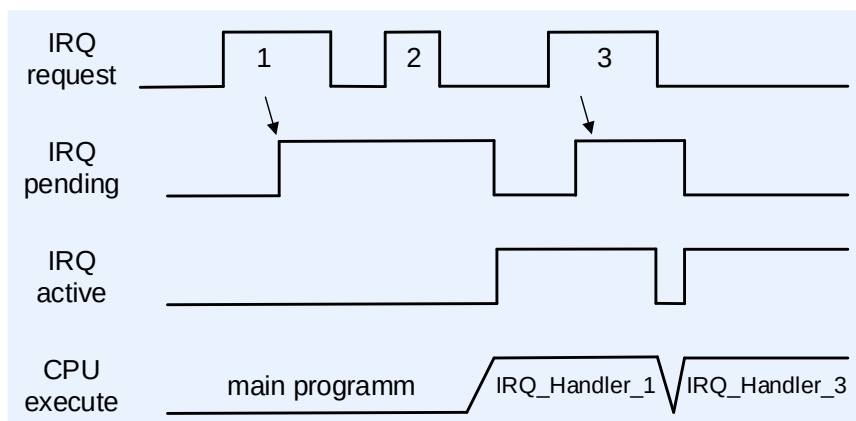
Рисунок 148 – Повторная установка запроса на прерывание в момент выполнения обработчика исключения
