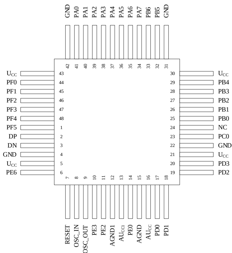
Рисунок 10 – Расположение выводов в 48-выводном корпусе H16.48-1B
