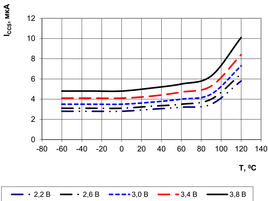
Рисунок 152 – Зависимость статического тока потребления в режиме покоя (регулятор напряжения выключен) от температуры при разном напряжении
