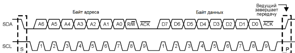
Рисунок 103 – Прием/передача по I2C в 7-битном режиме
