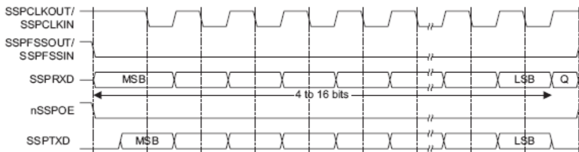
Рисунок 112 – Формат синхронного обмена протокола SPI, SPO=1, SPH=0 (одиночный обмен)
