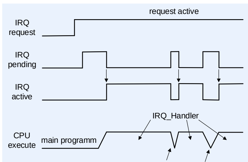
Рисунок 146 – Повторная обработка прерываний при удержании запроса от источника
