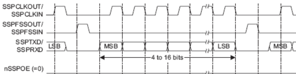
Рисунок 110 – Формат синхронного обмена протокола SPI, SPO=0, SPH=0 (непрерывный обмен)
