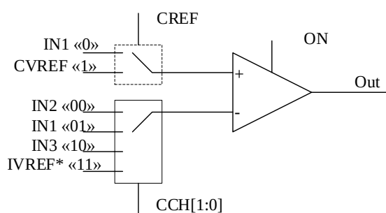
Рисунок 100 – Структура блока компаратора
