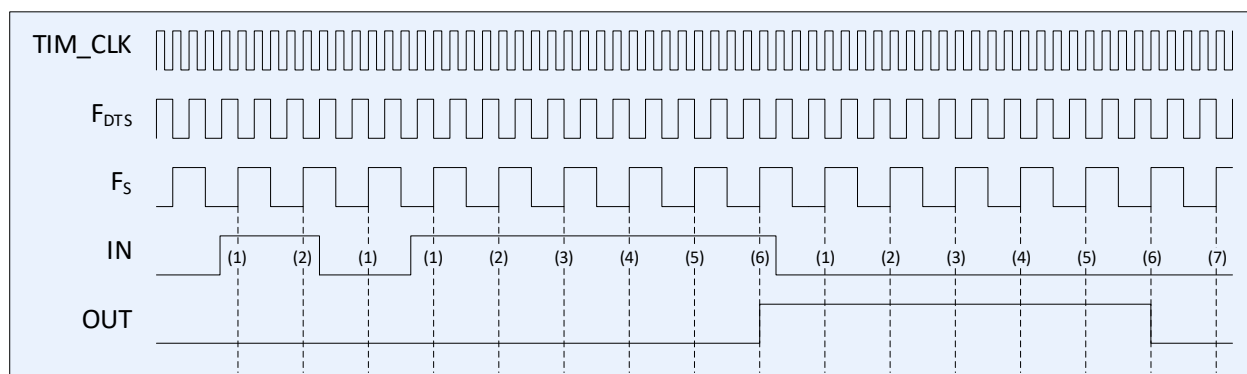
Рисунок 93 – Диаграмма работы фильтра, F_S = F_{DTS}/2 , N = 6
