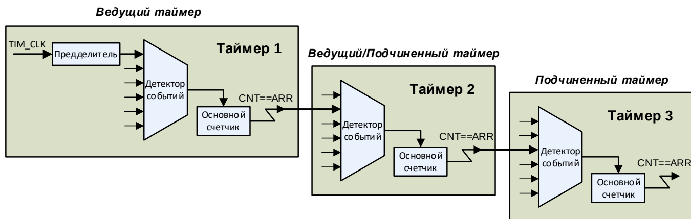
Рисунок 78 – Пример каскадного соединения таймеров
