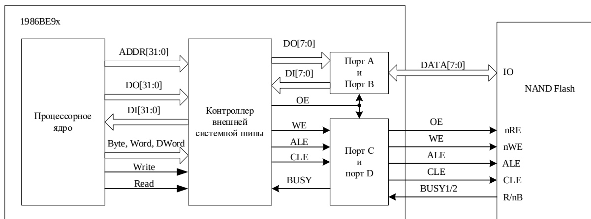
Рисунок 41 – Подключение внешней NAND Flash
