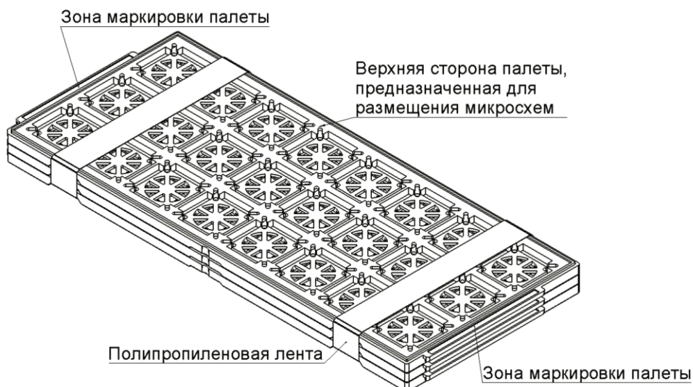
Рисунок 166 – Стопка палет
