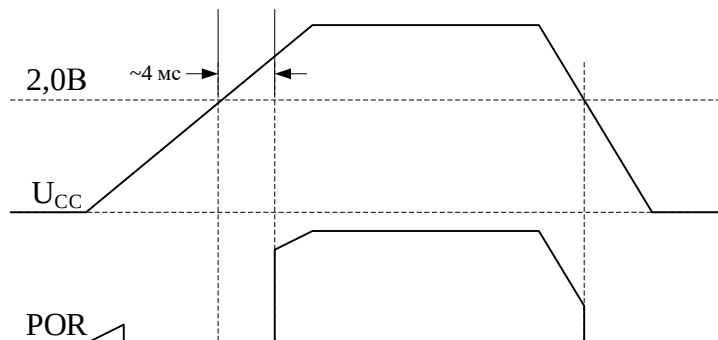
Рисунок 12 – Сигнал сброса при включении и выключении основного напряжения питания
