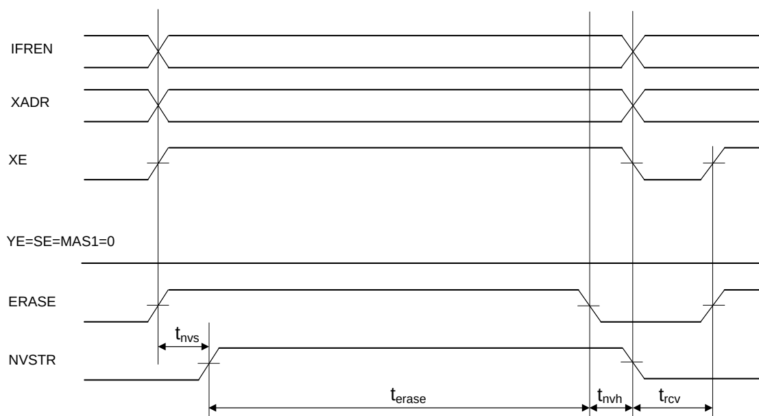
Рисунок 22 – Временная диаграмма стирания банка памяти
