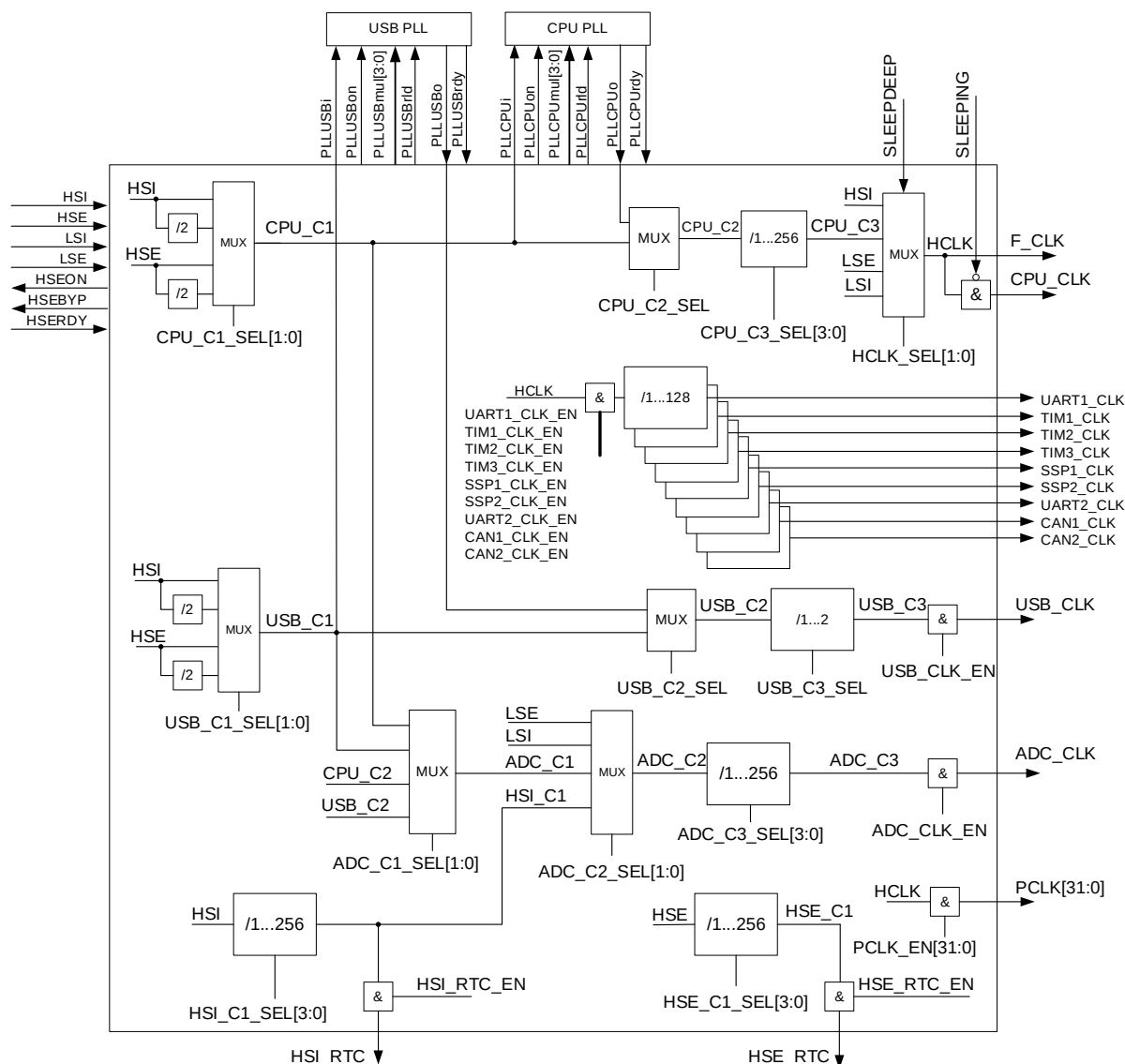
Рисунок 33 – Структурная блок-схема формирования тактовой частоты
