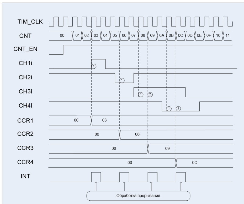
Рисунок 95 – Диаграммы примера работы в режиме захвата
