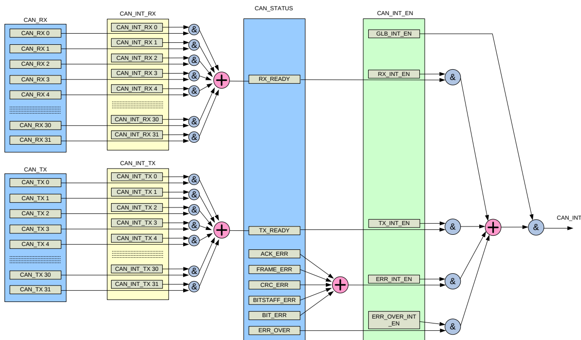
Рисунок 67 – Схема формирования прерывания блока CAN
