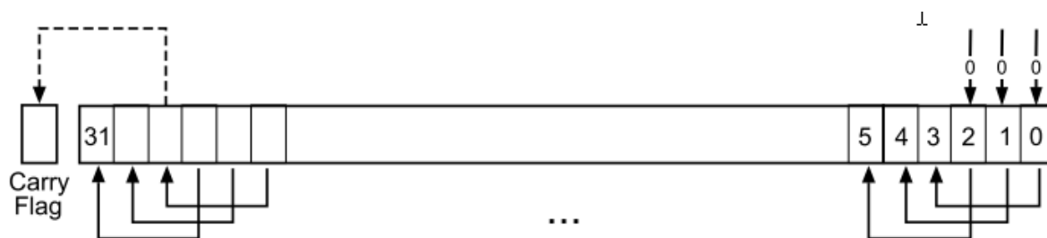
Рисунок 29 – Инструкция LSL # 3
