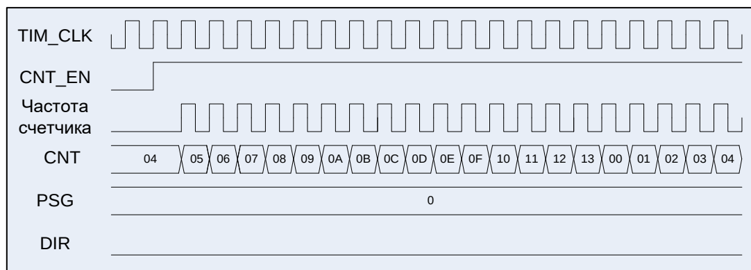
Рисунок 69 – Диаграммы работы таймера, счет прямой от 0 до 0x13, стартовое значение 0x04
