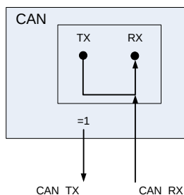
Рисунок 52 – Режим работы только на прием - Receive Only Mode
