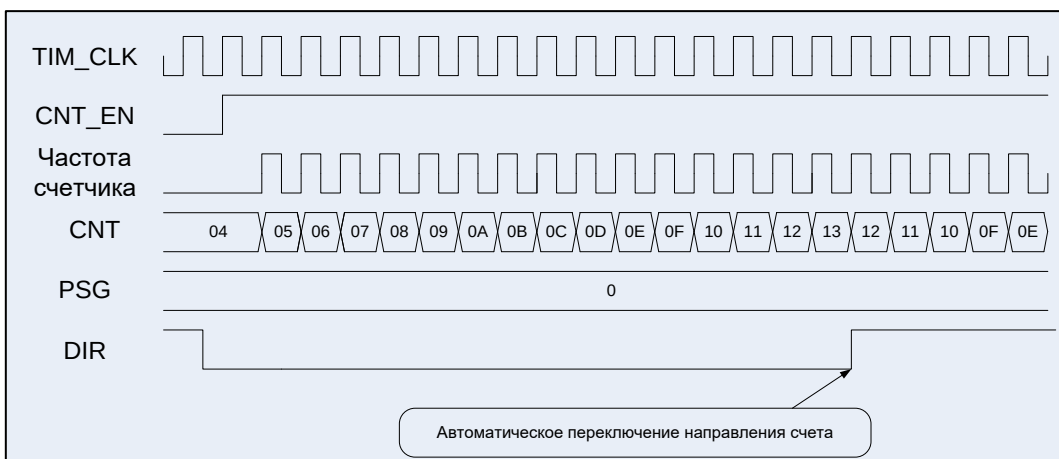
Рисунок 71 – Диаграммы работы таймера, счет двунаправленный, сначала прямой
