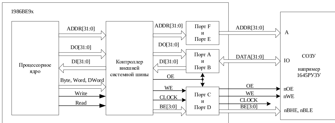
Рисунок 42 – Обмен по внешней системной шине при задании длительности через биты WAIT_STATE
