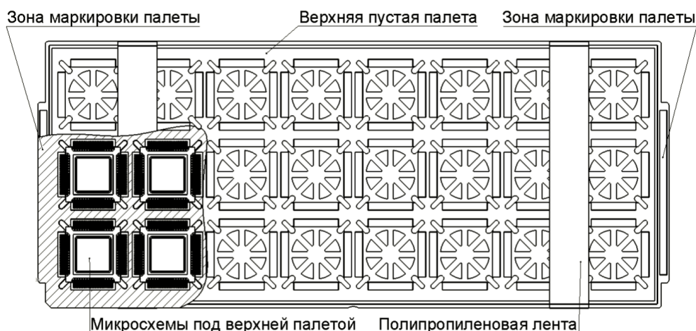
Рисунок 167 – Стопка палет. Вид сверху
