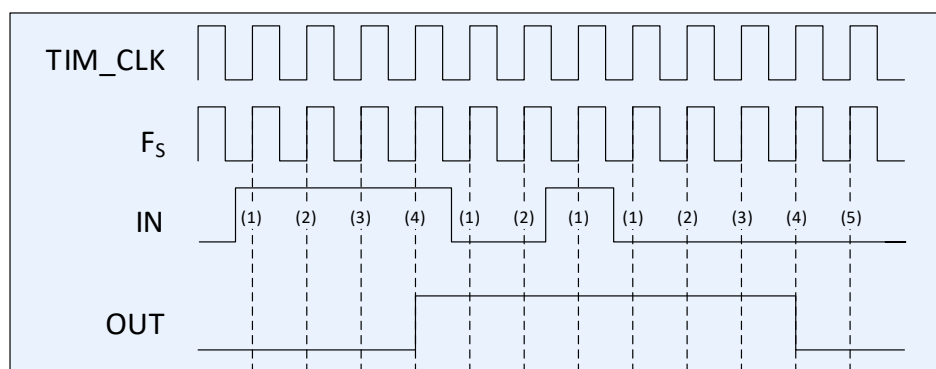
Рисунок 92 – Диаграмма работы фильтра, F_S = \text{TIM\_CLK} , N = 4
