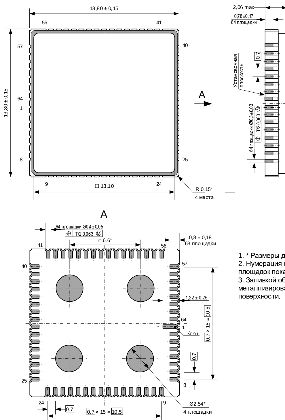
Рисунок 161 – Корпус МК 5153.64-2
