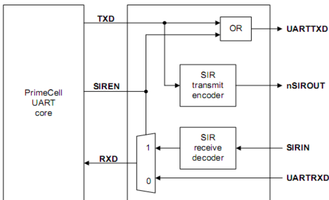
Рисунок 123 – Структурная схема кодека IrDA
