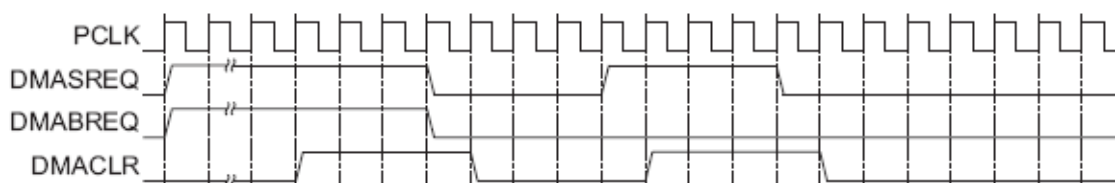
Рисунок 121 – Временные диаграммы обмена в режиме DMA
