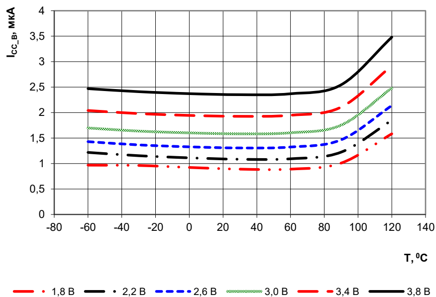
Рисунок 153 – Зависимость тока потребления батарейного домена от температуры при разном напряжении
