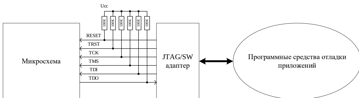
Рисунок 19 – Схема работы в режиме отладки
