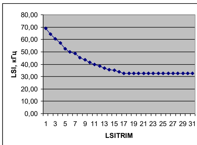
Рисунок 35 – Зависимость частоты LSI от значения LSITRIM
