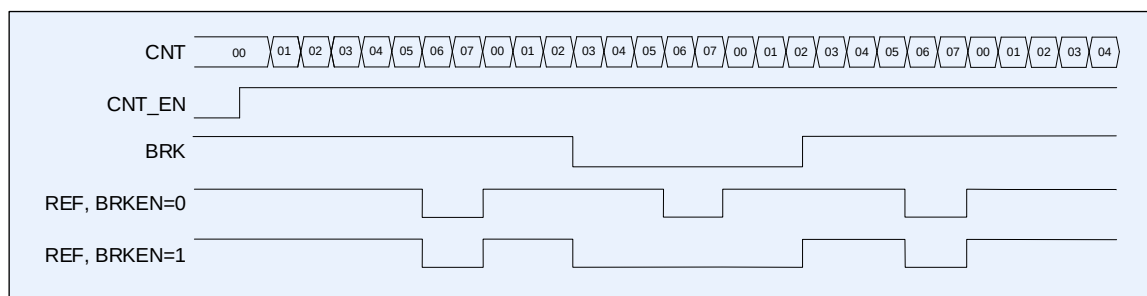
Рисунок 90 – Диаграмма сброса сигнала REF по выводу BRK
