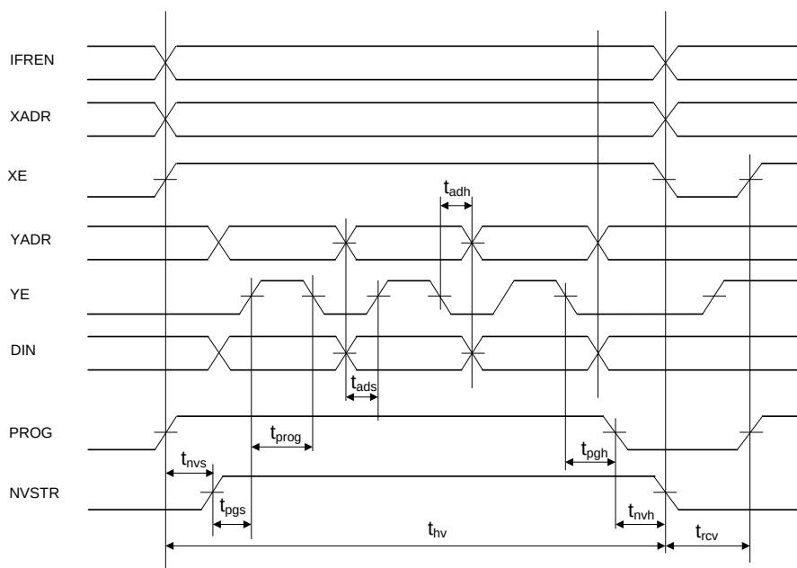
Рисунок 23 – Временная диаграмма записи памяти
