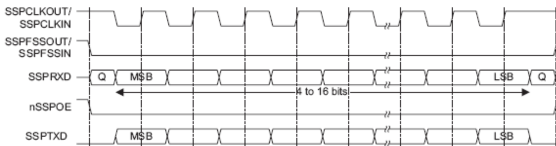
Рисунок 114 – Формат синхронного обмена протокола SPI, SPO=1, SPH=1
