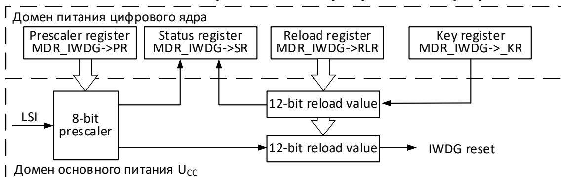
Рисунок 149 – Блок-схема независимого сторожевого таймера
