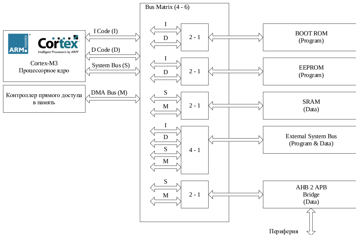
Рисунок 15 – Структурная схема организации памяти
