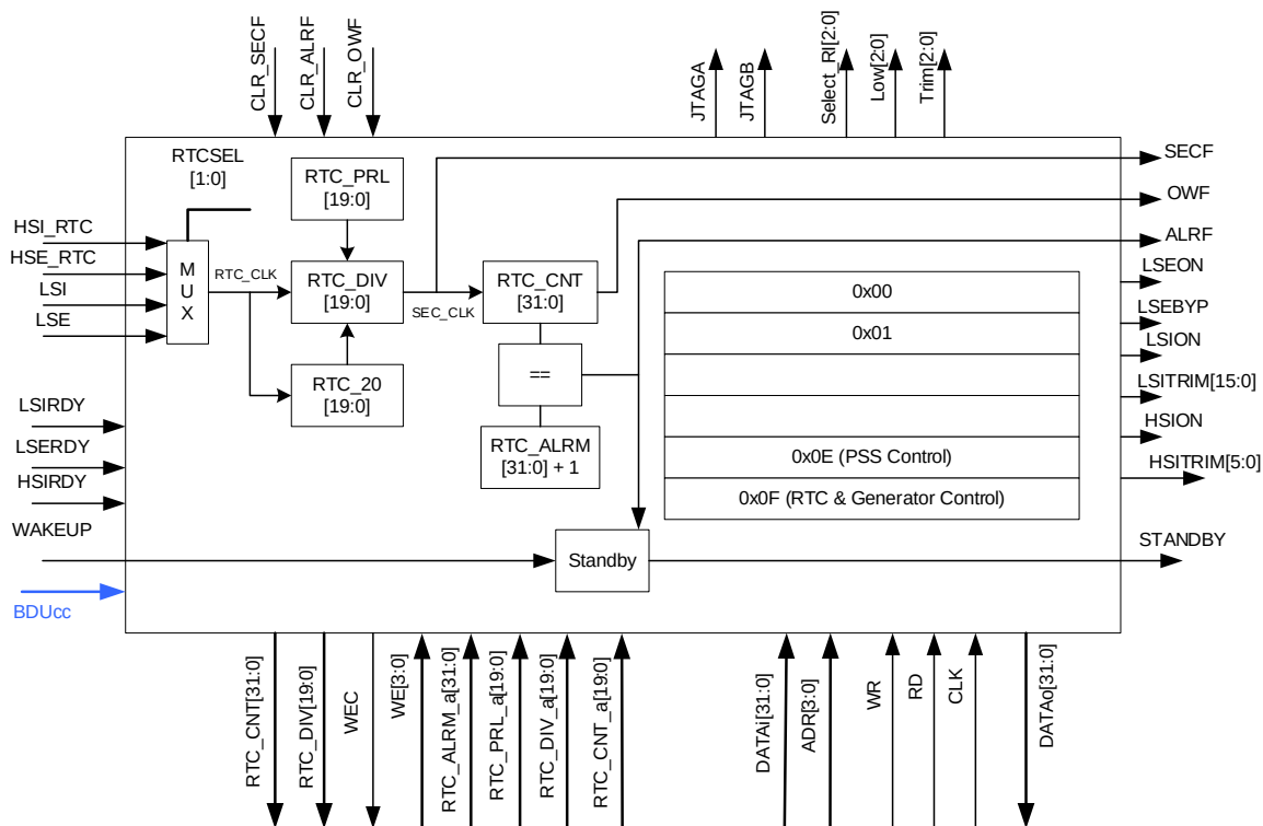
Рисунок 34 – Структурная блок-схема батарейного домена и часов реального времени
