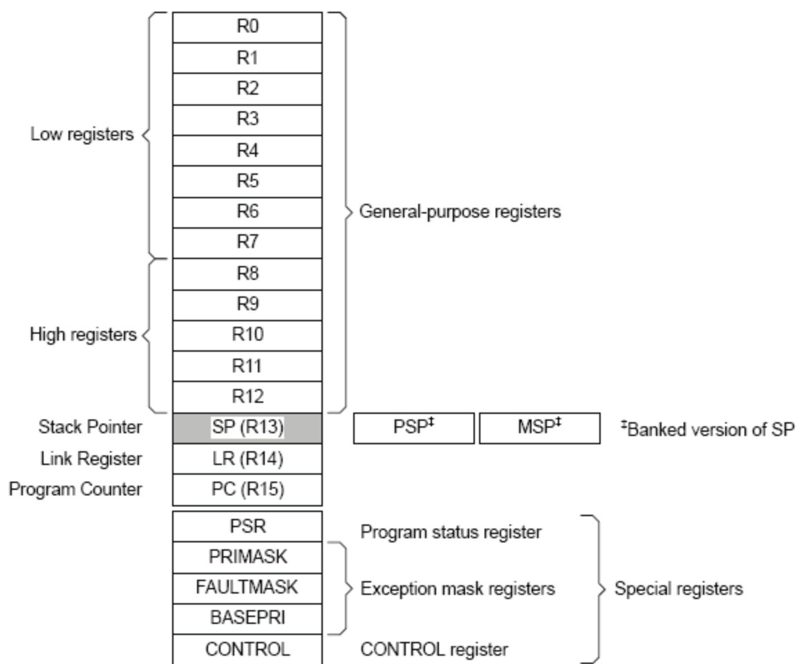
Рисунок 26 – Регистры ядра
