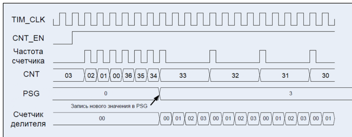
Рисунок 77 – Диаграмма работы счетчика: счет обратный (CNT_MODE[1:0] = 00, EVENT_SEL[3:0] = 0000, DIR = 1)
