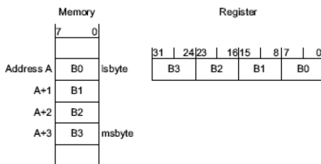
Рисунок 18 – Организация расположения байтов в 32-битной памяти
