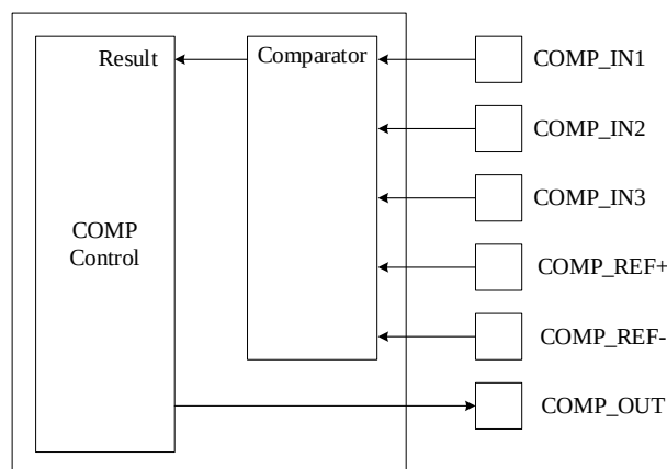
Рисунок 100 – Структура блока компаратора
