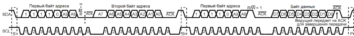
Рисунок 104 – Прием по I2C в 10-битном режиме
