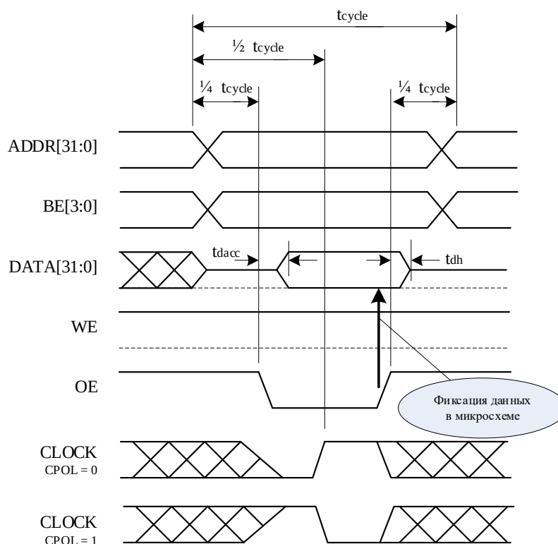
Рисунок 44 – Диаграмма чтения
