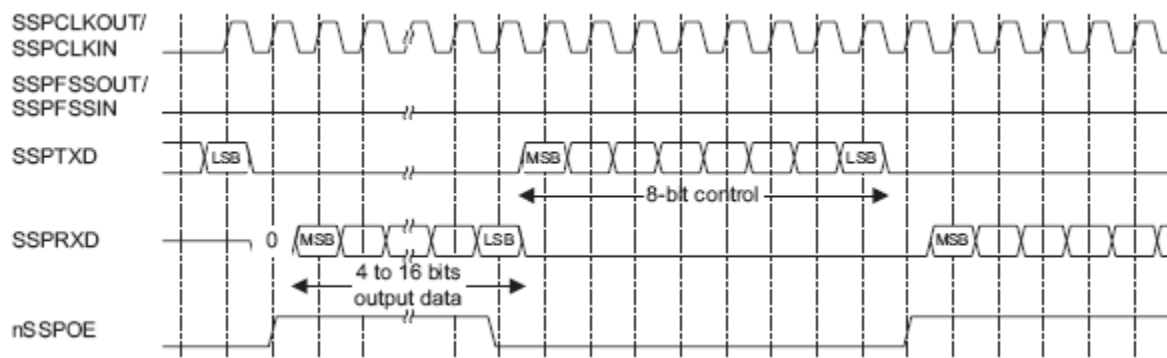
Рисунок 116 – Формат синхронного обмена протокола Microwire (непрерывный обмен)
