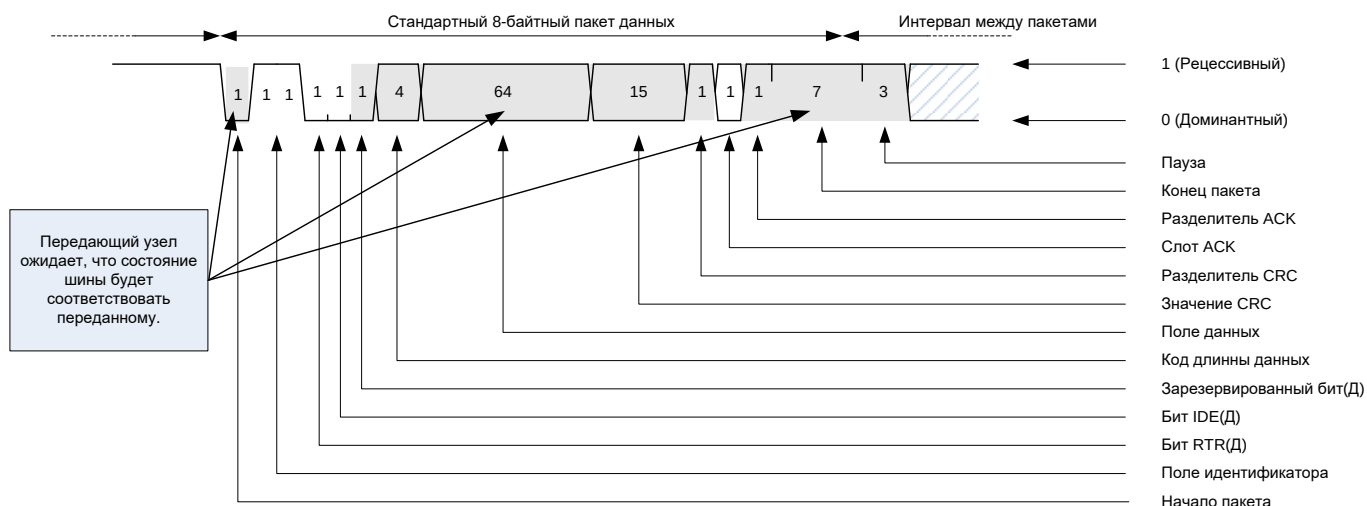
Рисунок 64 – Контроль передаваемых бит
