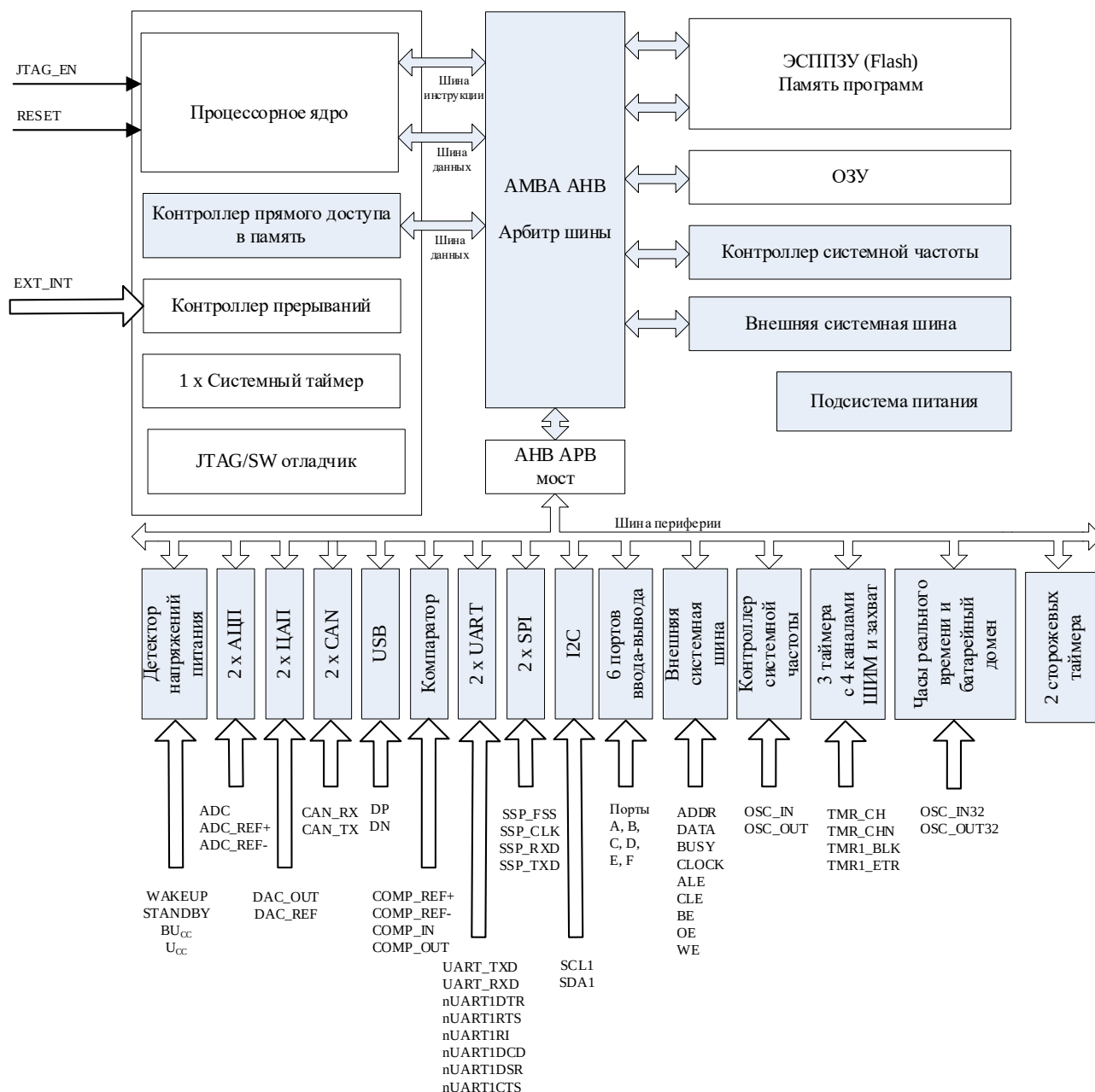
Рисунок 1 – Структурная блок-схема микросхем K1986BE91T, K1986BE94T, K1986BE94Ф, K1986BE94Я
