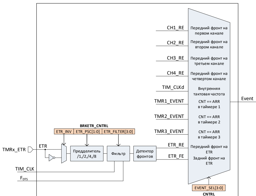
Рисунок 82 – Схема тактирования сигналом со входа ETR
