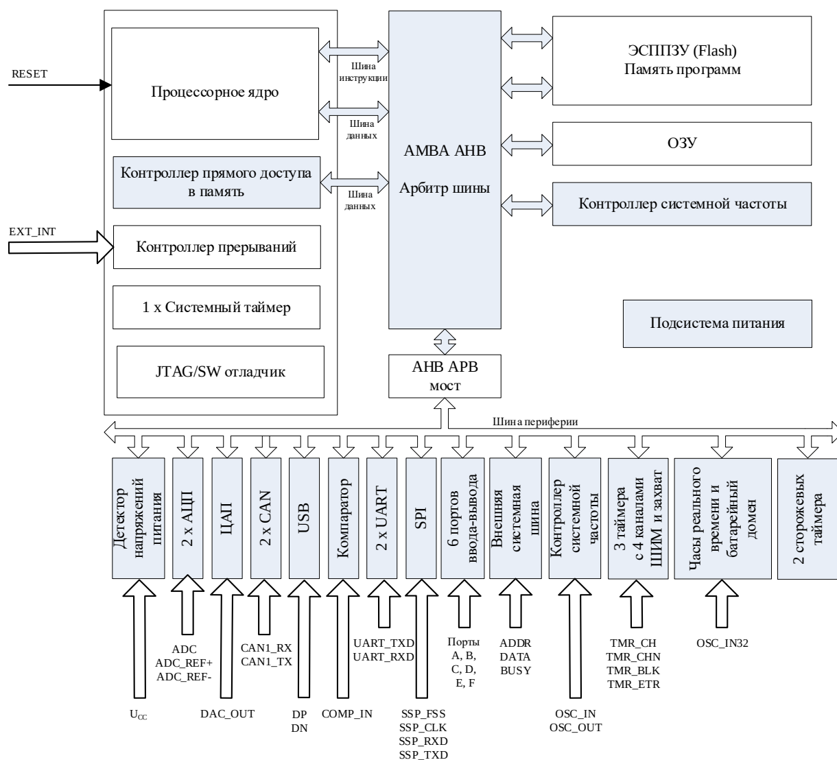
Рисунок 3 – Структурная блок-схема микросхем K1986BE93У
