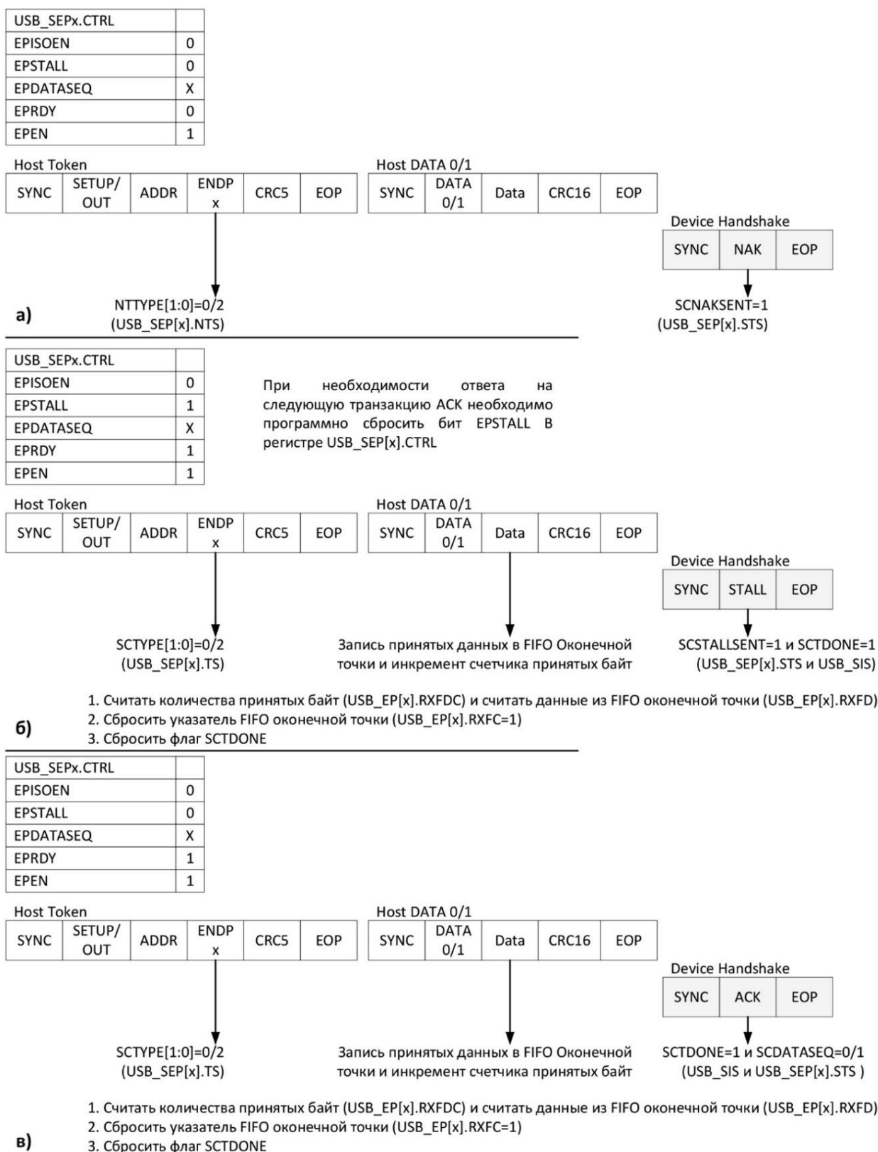
Рисунок 47 – Транзакция SETUP/OUT (USB Device)
