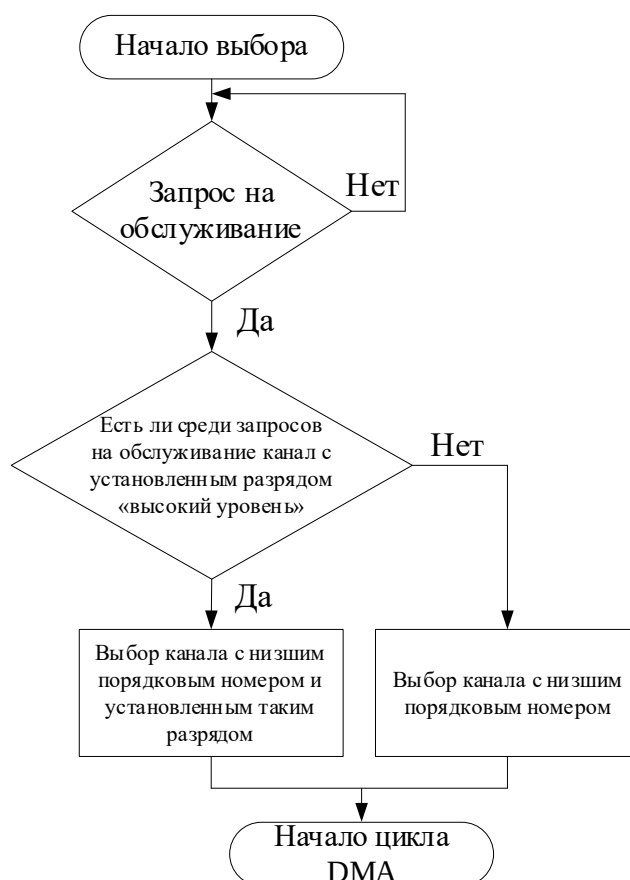
Рисунок 135 – Алгоритм выбора следующего канала для обслуживания
