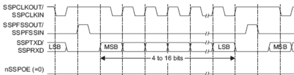
Рисунок 113 – Формат синхронного обмена протокола SPI, SPO=1, SPH=0 (непрерывный обмен)
