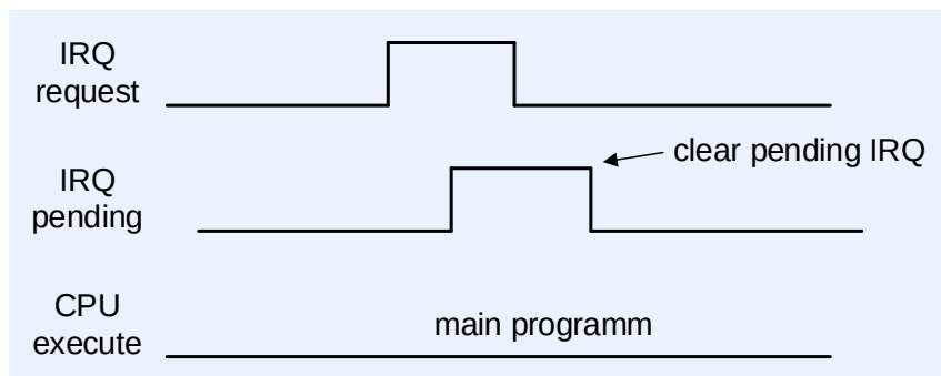
Рисунок 144 – Сброс признака отложенного прерывания, до обработки ядром
