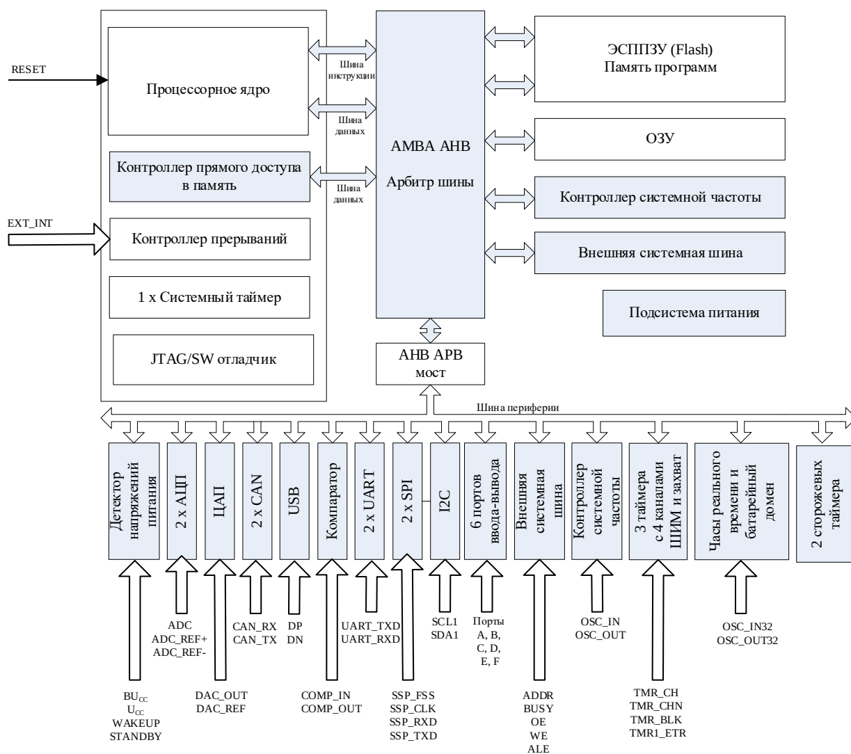
Рисунок 2 – Структурная блок-схема микросхем K1986BE92У, K1986BE92У1
