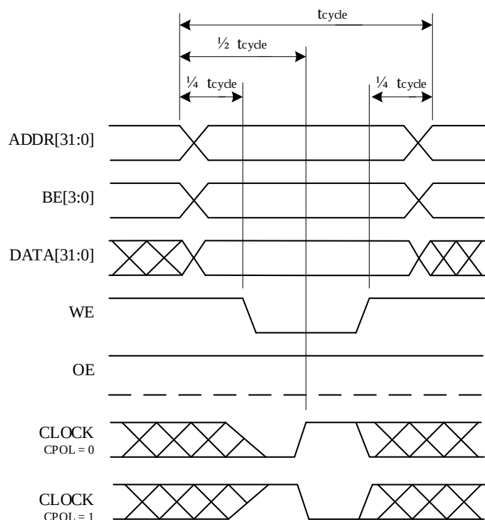
Рисунок 43 – Диаграмма записи
