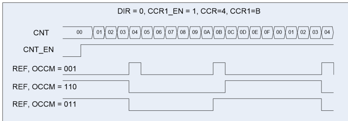
Рисунок 88 – Диаграмма работы в режиме ШИМ, CCR1_EN = 1
