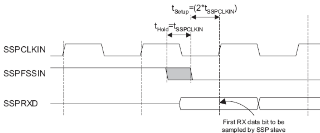
Рисунок 117 – Формат Microwire, требования к времени установки и удержания сигнала
