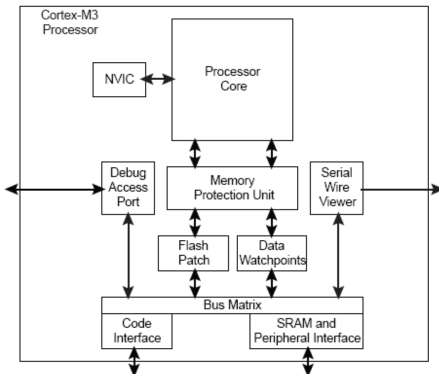
Рисунок 25 – Структурная блок-схема процессорного ядра Cortex-M3
