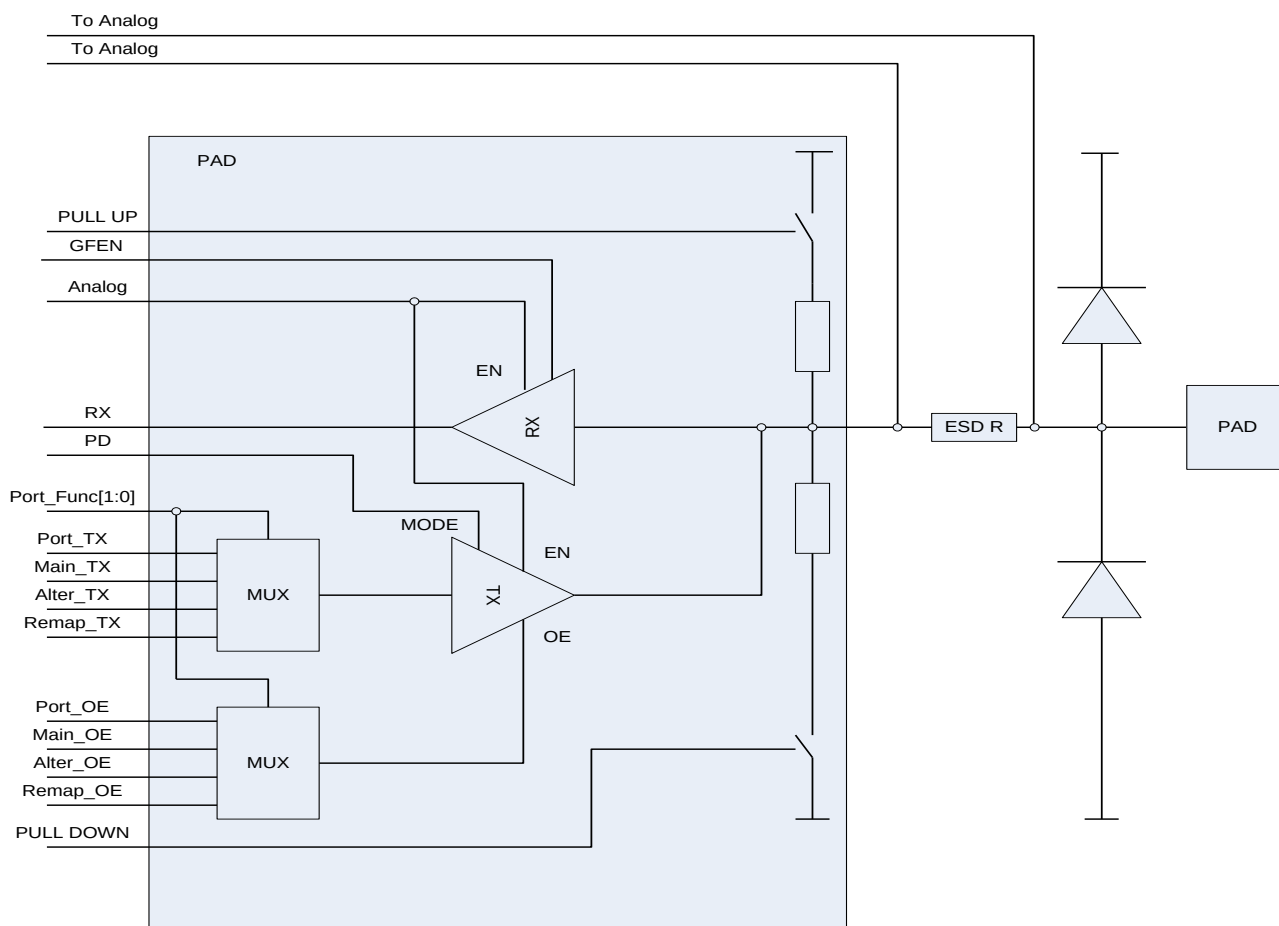
Рисунок 37 – Порты ввода-вывода
