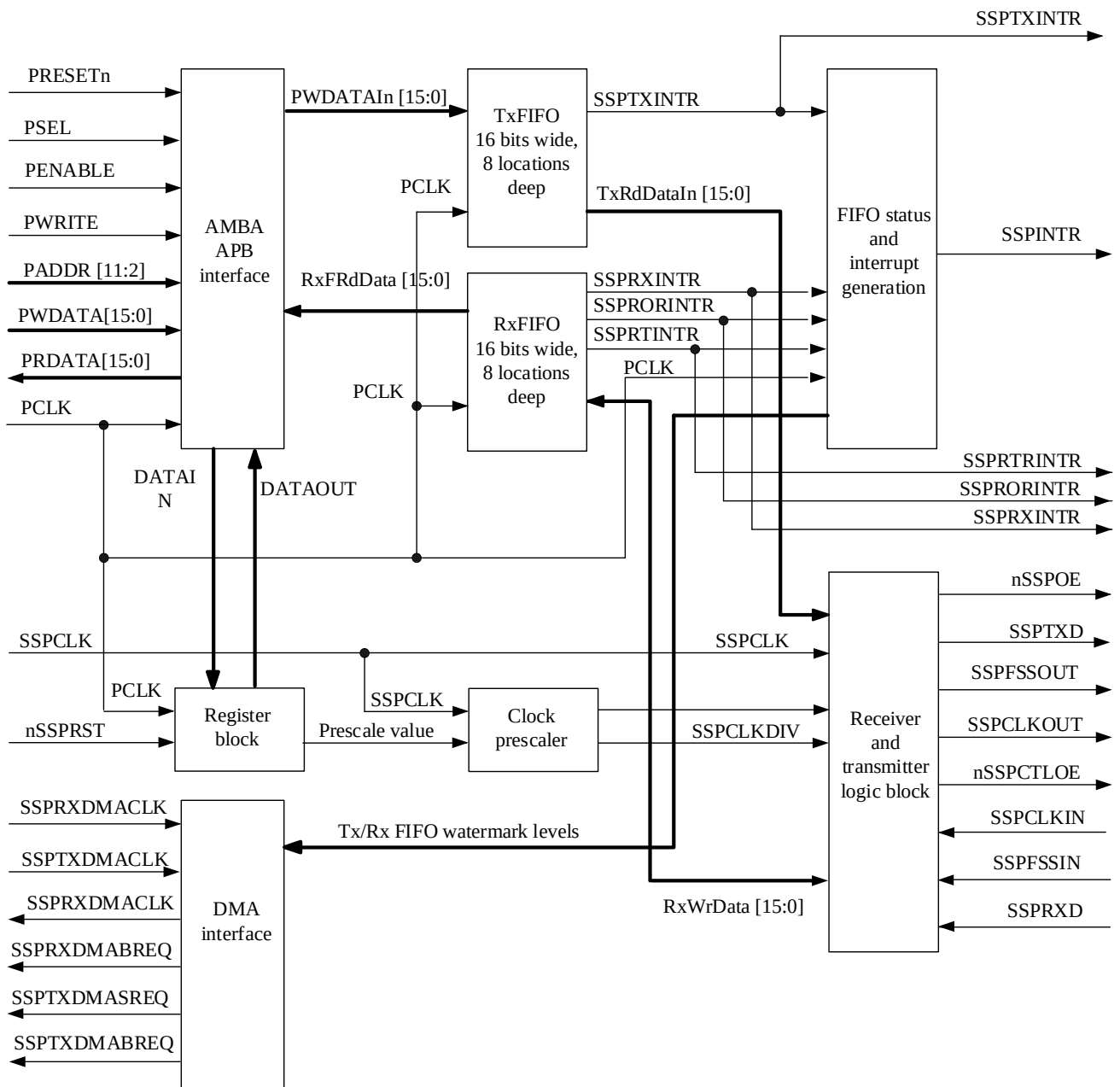
Рисунок 106 – Структурная схема модуля SSP
