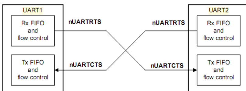
Рисунок 127 – Взаимодействие двух устройств последовательной связи с аппаратным управлением потоком данных
