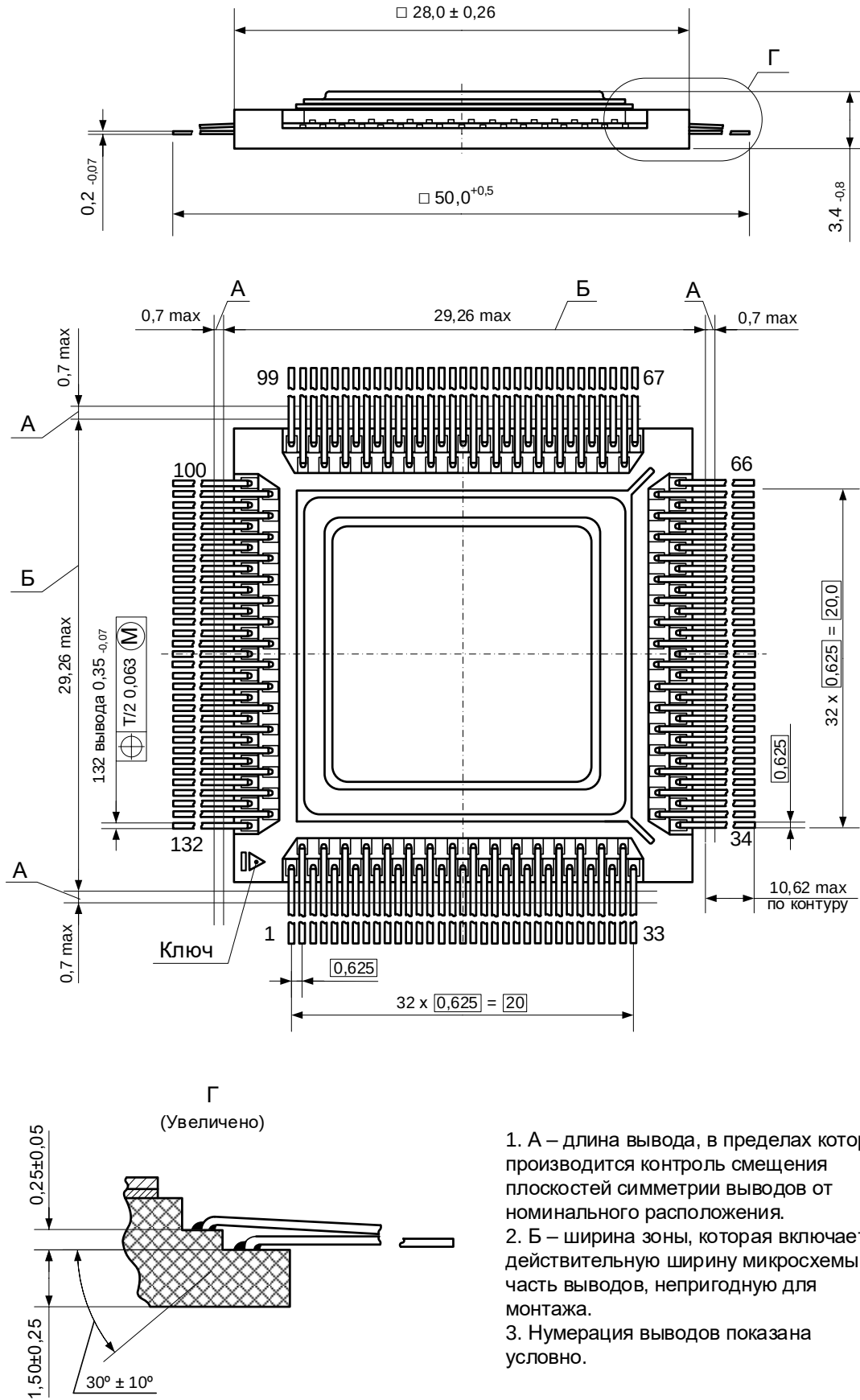
Рисунок 158 – Габаритный чертеж микросхемы в корпусе 4229.132-3
