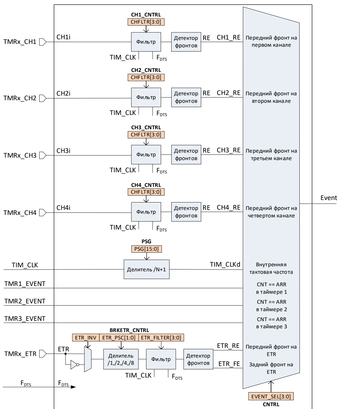
Рисунок 75 – Структурная схема формирования события для счета
