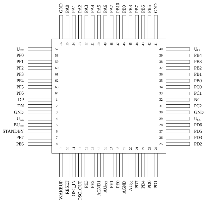
Рисунок 9 – Расположение выводов в 64-выводном корпусе H18.64-1B
