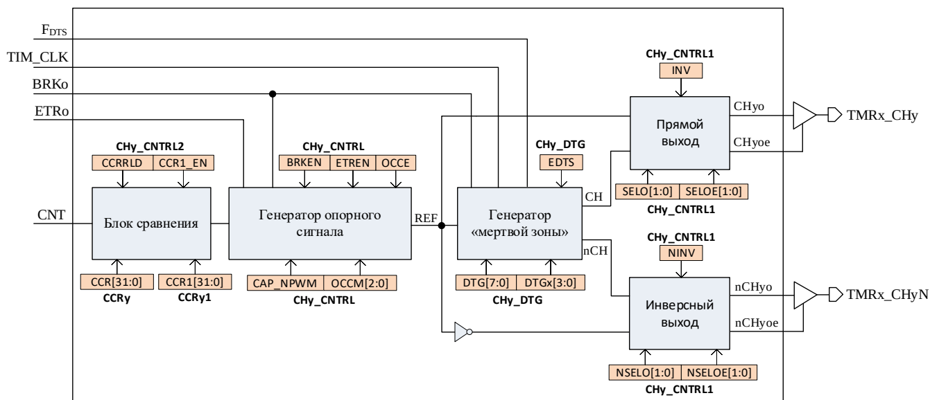
Рисунок 86 – Структурная схема блока формирования ШИМ
