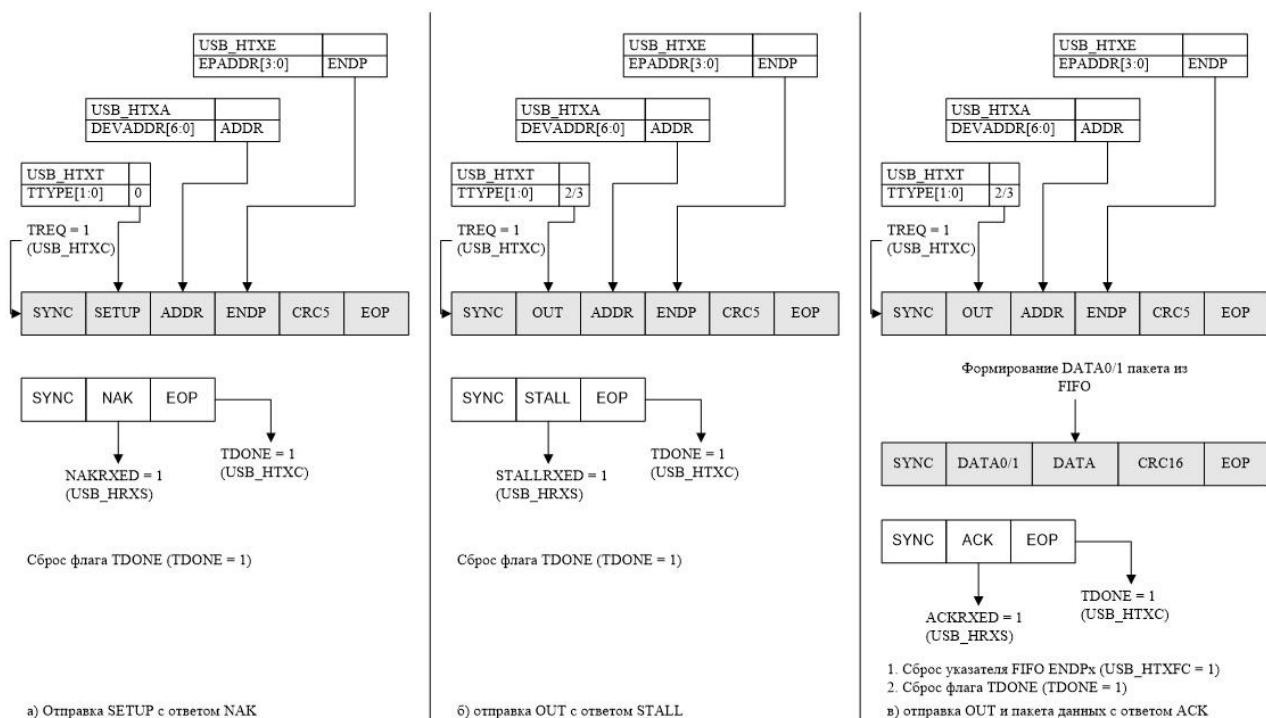
Рисунок 48 (а, б, в) – Транзакция SETUP/OUT (USB Host)
