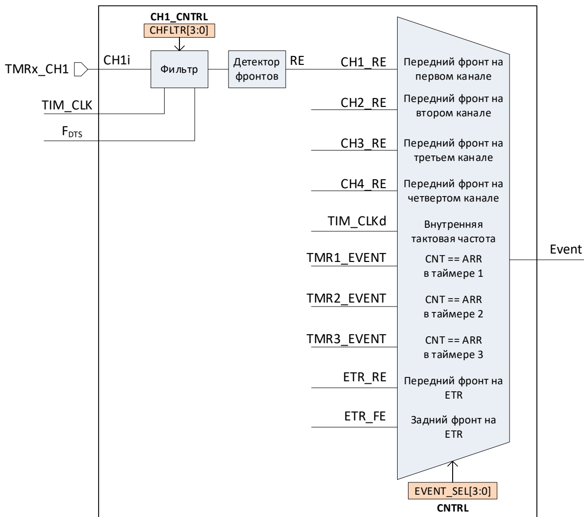
Рисунок 80 – Схема тактирования сигналом со входа первого канала
