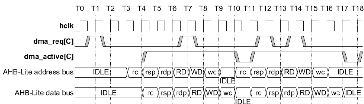
Рисунок 130 – Диаграмма работы при получении импульсного запроса
