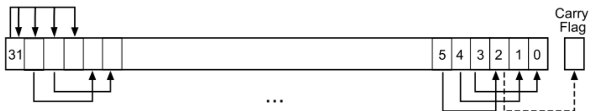
Рисунок 27 – Инструкция ASR # 3
