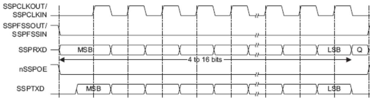
Рисунок 109 – Формат синхронного обмена протокола SPI, SPO=0, SPH=0 (одиночный обмен)
