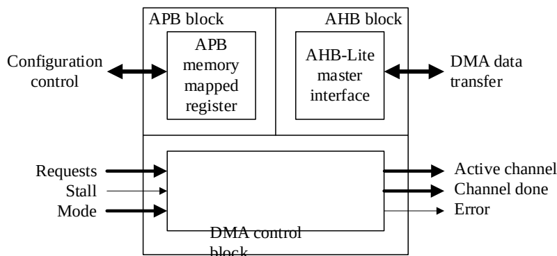
Рисунок 129 – Структурная схема контроллера
