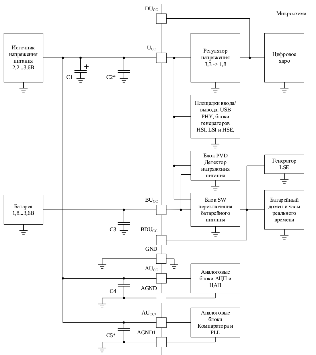
Рисунок 11 – Структурная блок-схема подачи питания
