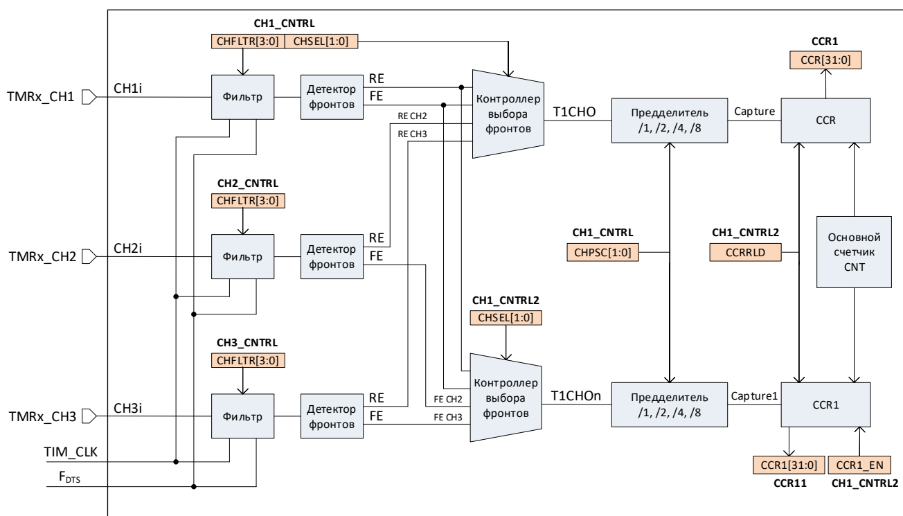
Рисунок 84 – Структурная схема блока захвата на примере канала 1
