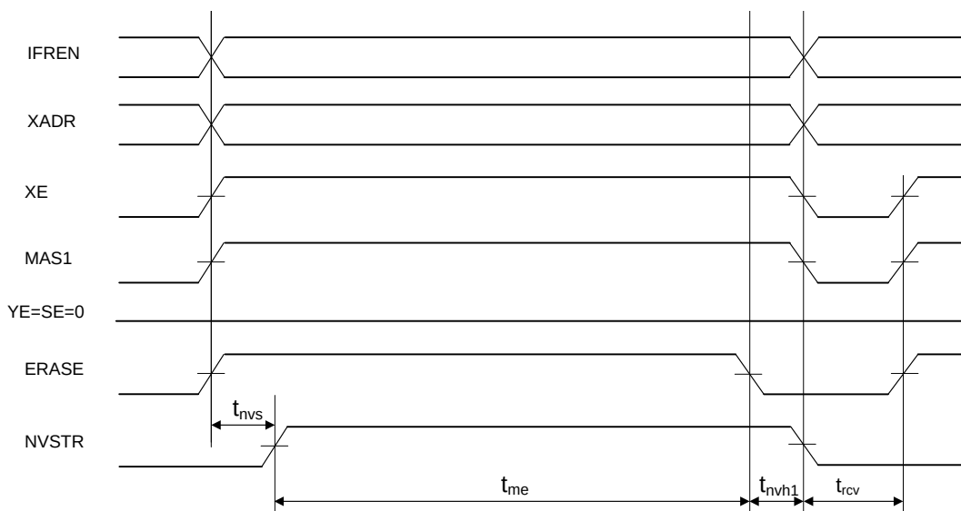
Рисунок 21 – Временная диаграмма стирания памяти
