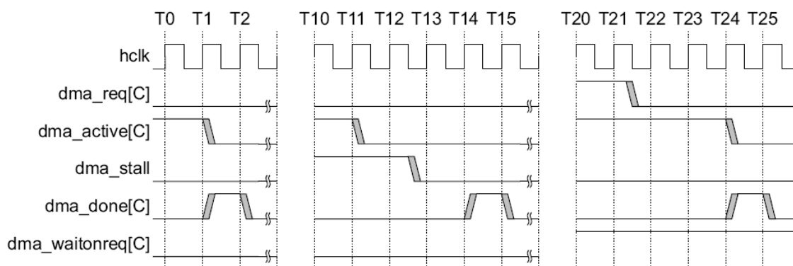
Рисунок 132 – Диаграммы функционирования dma_done
