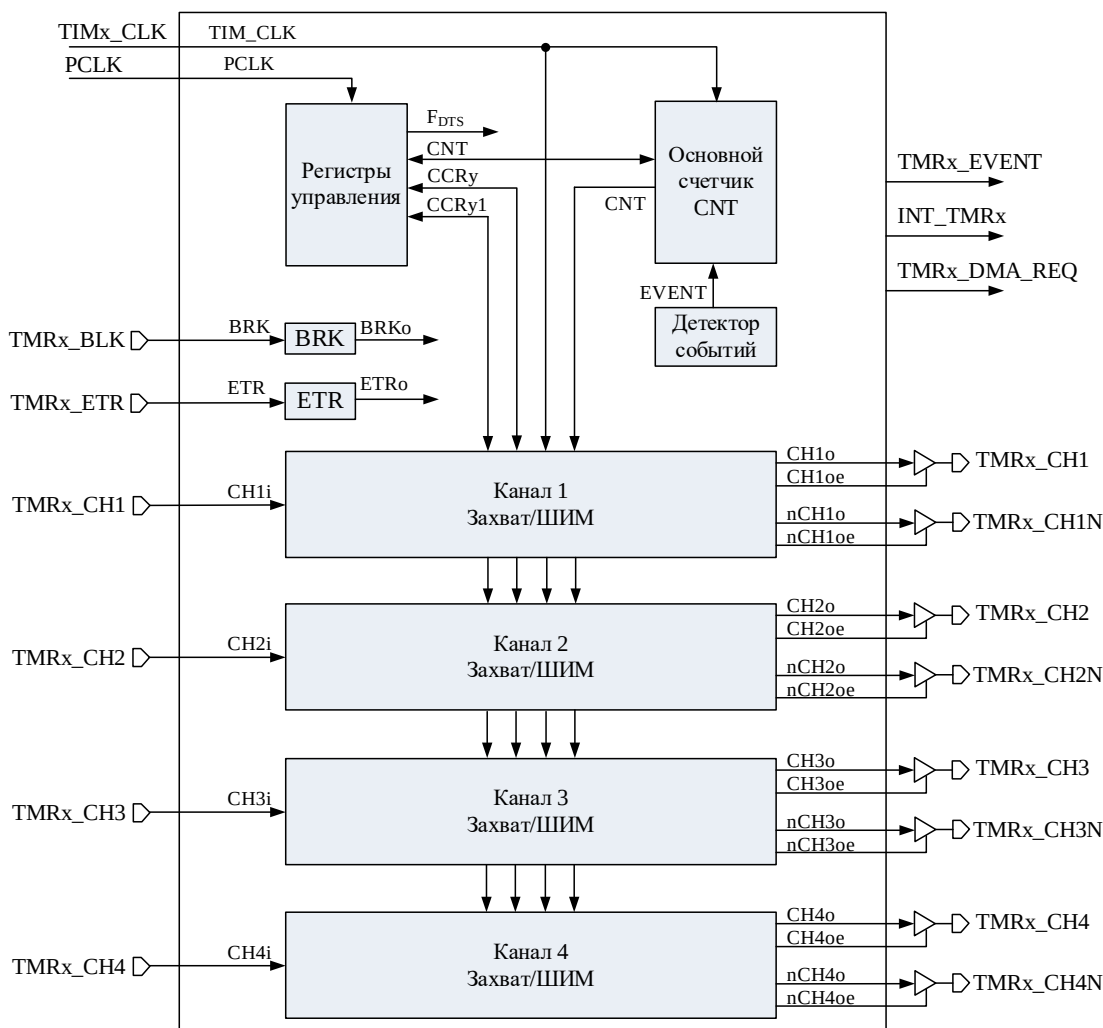
Рисунок 68 – Структурная схема блока «Таймер»
