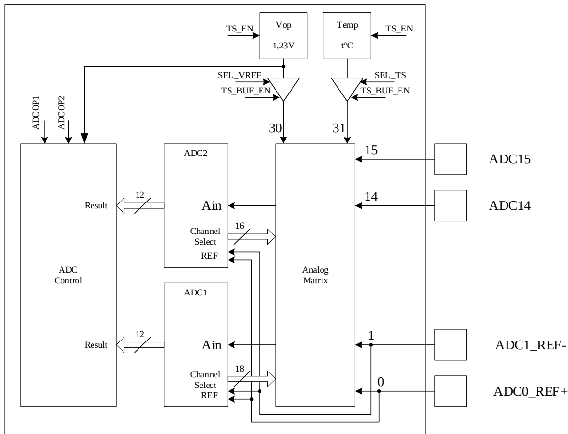
Рисунок 97 – Структурная схема контроллера АЦП
