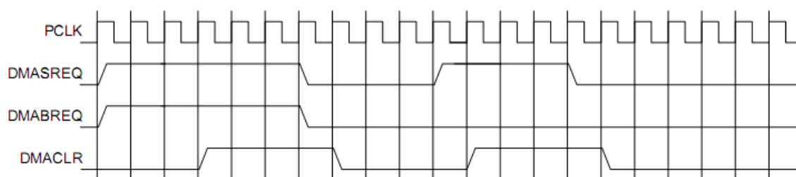
Рисунок 128 – Временные диаграммы одноэлементного и блочного запросов DMA
