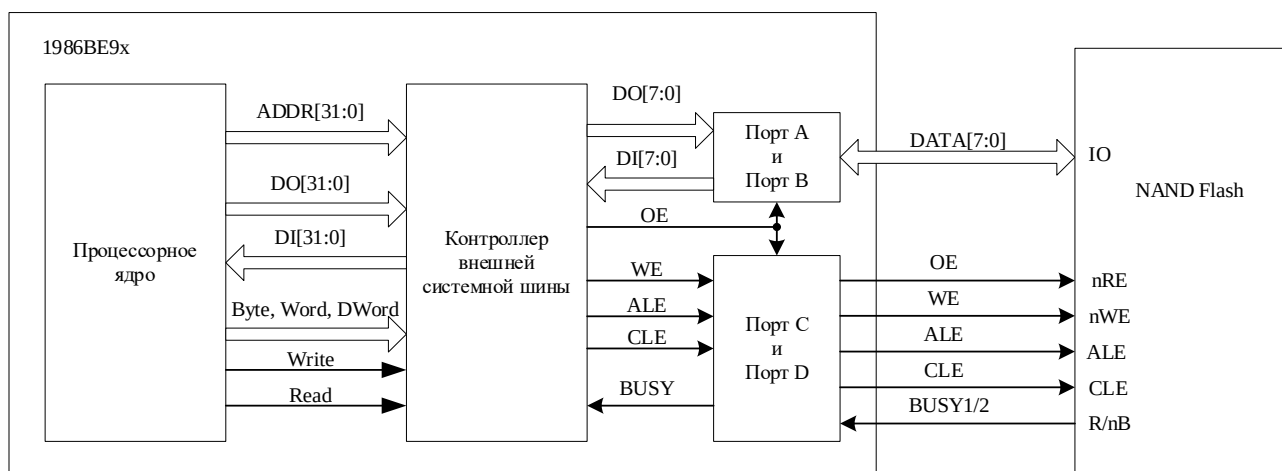
Рисунок 45 – Подключение внешней NAND Flash
