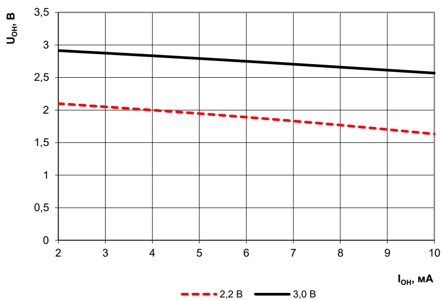
Рисунок 155 – Зависимость выходного напряжения высокого уровня от выходного тока высокого уровня при напряжении питания 2,2 и 3,0 В
