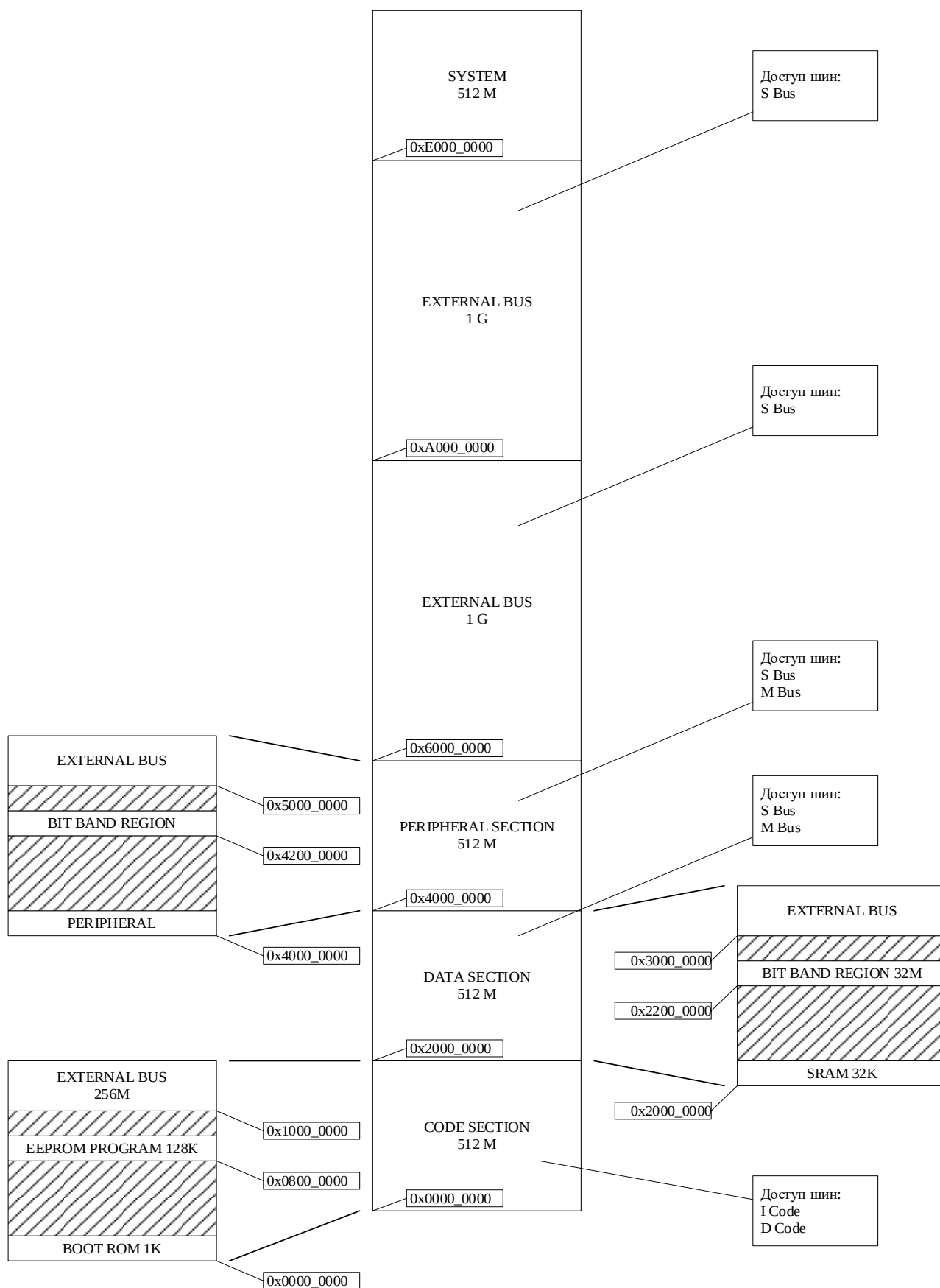
Рисунок 16 – Карта распределения основных областей памяти
