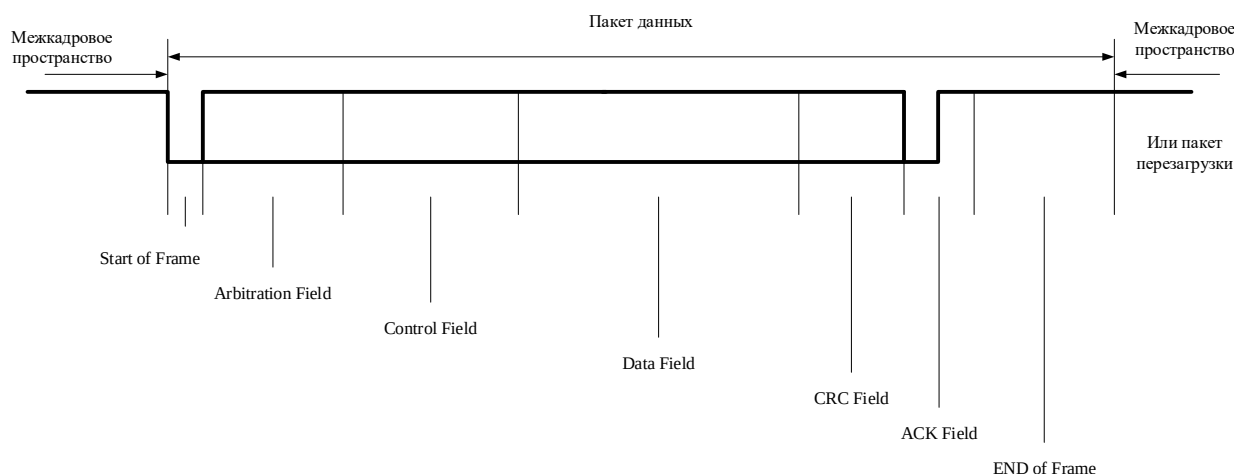
Рисунок 55 – Пакет сообщения CAN
