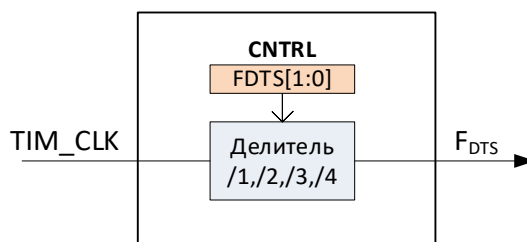
Рисунок 73 – Схема формирования тактовой частоты F_{DTS}
