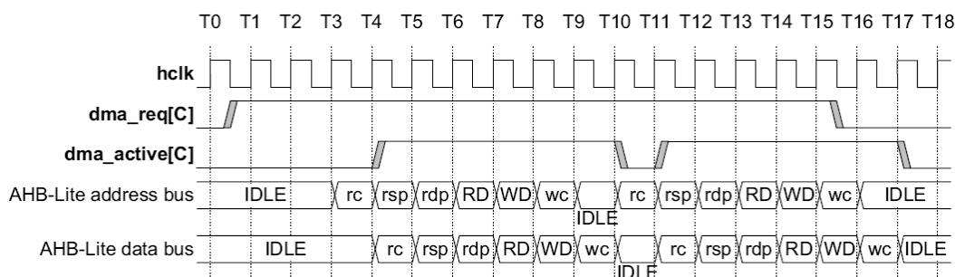
Рисунок 131 – Диаграмма работы при получении запроса на обработку по уровню.
