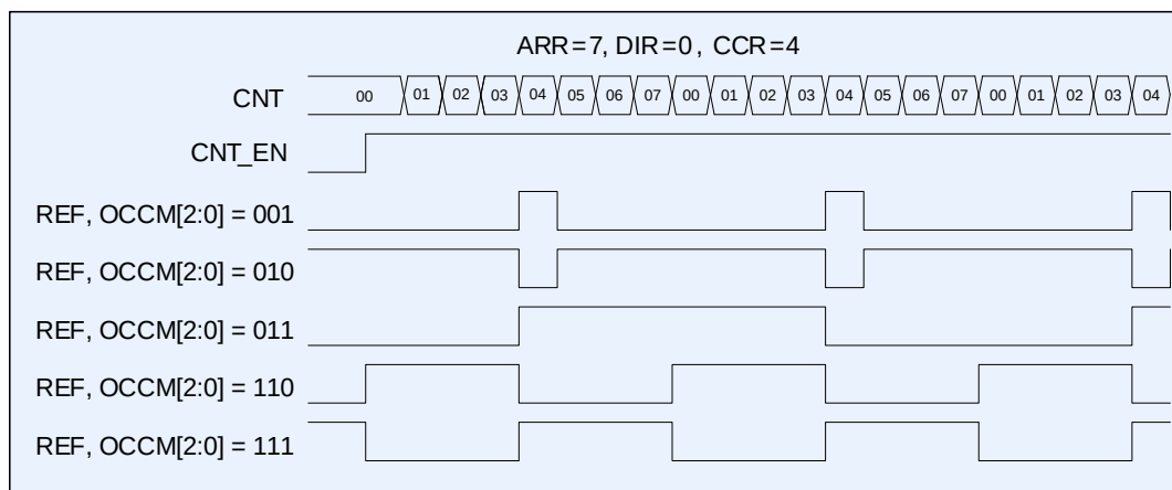
Рисунок 87 – Диаграмма работы в режиме ШИМ, CCR1_EN=0
