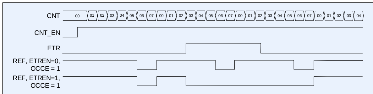
Рисунок 89 – Диаграмма сброса сигнала REF по выводу ETR
