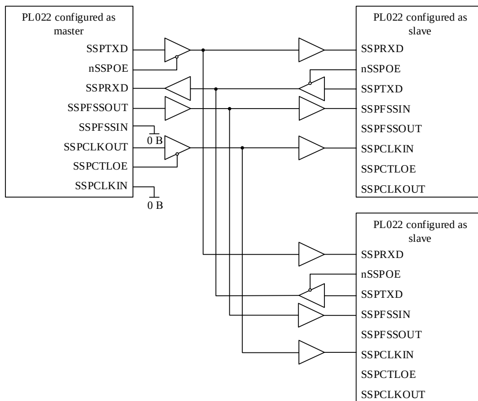
Рисунок 118 – Ведущее устройство SSP подключено к двум ведомым
