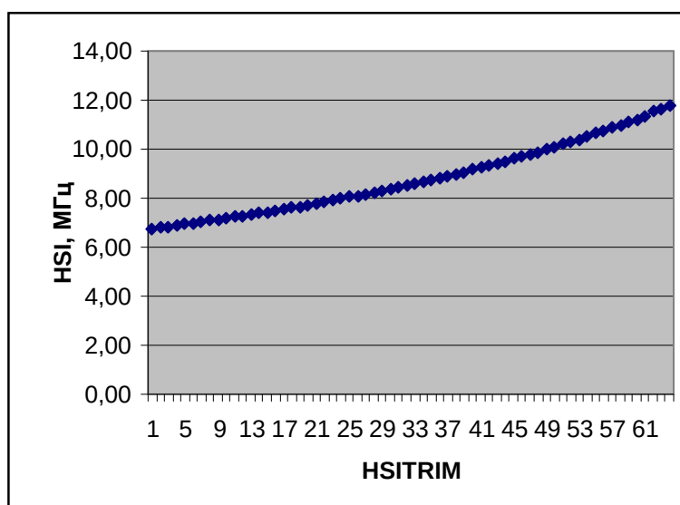
Рисунок 36 – Зависимость частоты HSI от значения HSITRIM
