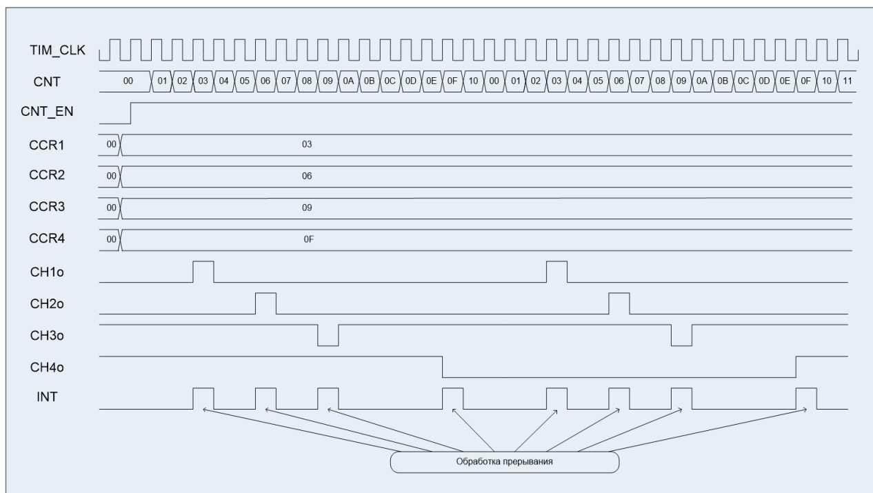
Рисунок 96 – Диаграммы примера работы в режиме ШИМ
