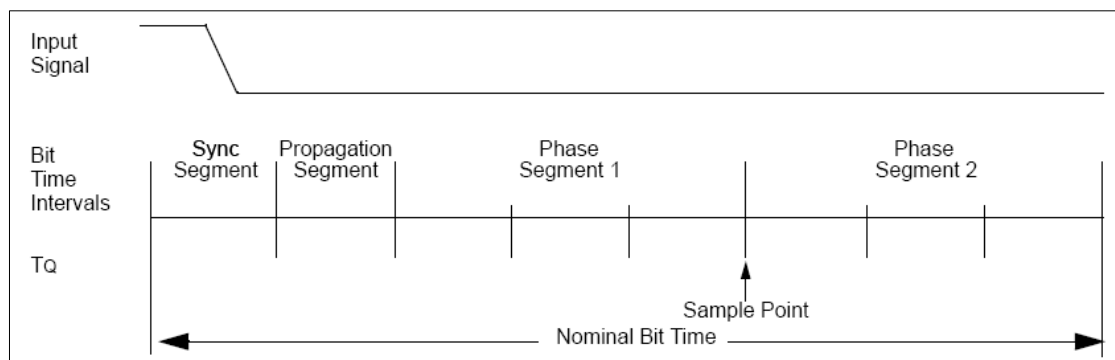
Рисунок 60 – Структура битового интервала
