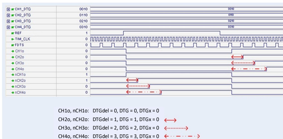
Рисунок 91 – Диаграмма работы блока DTG
