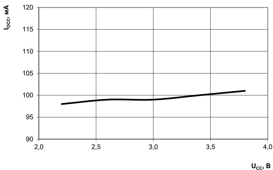
Рисунок 151 – Зависимость динамического тока потребления от напряжения питания
