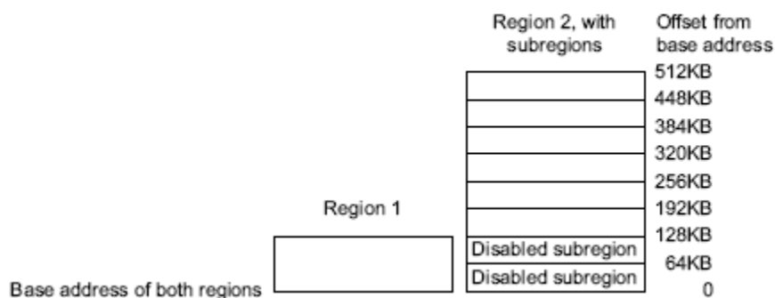
Рисунок 32 – Применение SRD
