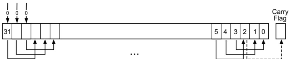
Рисунок 28 – Инструкция LSR # 3
