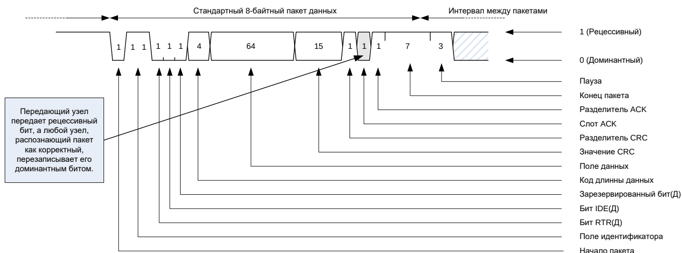
Рисунок 62 – Контроль подтверждения
