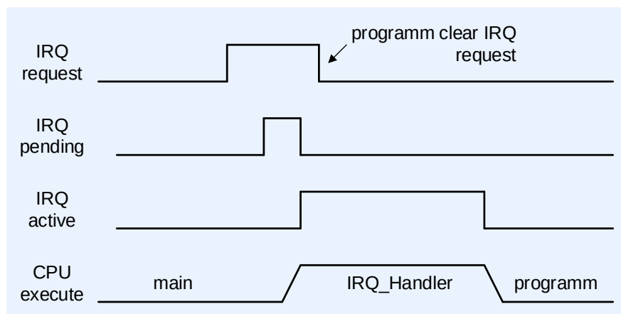
Рисунок 145 – Сброс признака отложенного прерывания, до обработки ядром
