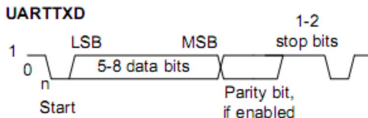
Рисунок 125 – Кадр передачи данных
