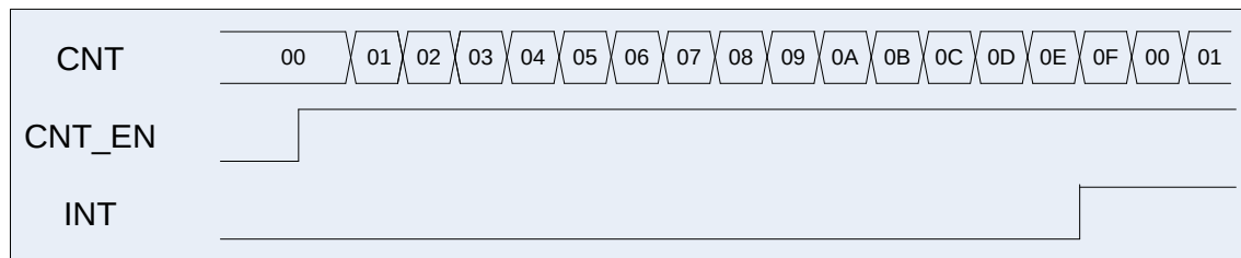
Рисунок 94 – Режим обычного счетчика
