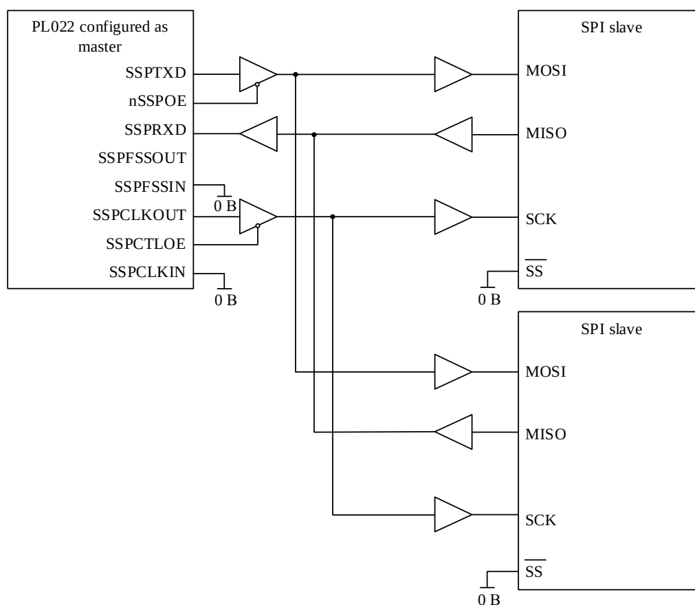
Рисунок 119 – Ведущее устройство SSP подключено к двум ведомым, поддерживающим SPI
