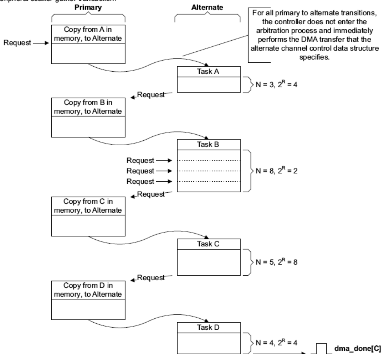
Рисунок 138 – Пример работы DMA в режиме с «Исполнением с изменением конфигурации»
