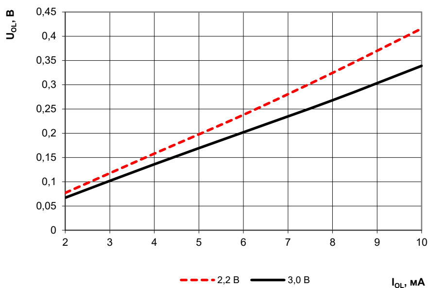
Рисунок 156 – Зависимость выходного напряжения низкого уровня от выходного тока низкого уровня при напряжении питания 2,2 и 3,0 В
