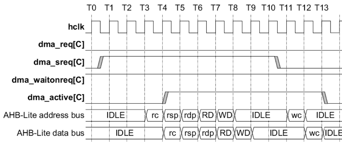
Рисунок 134 – Работа DMA при использовании dma_waitonreq совместно с dma_sreq
