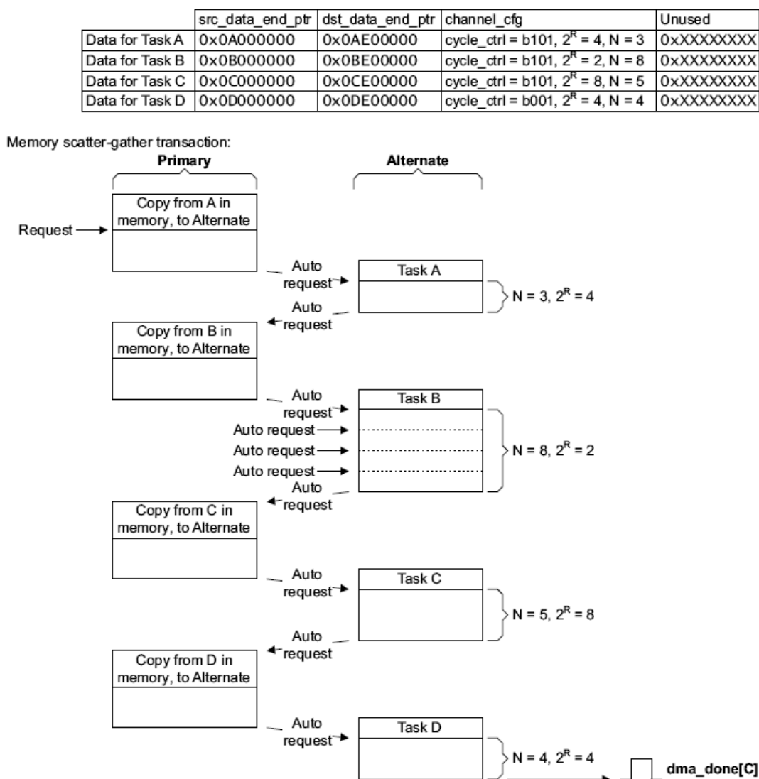
Рисунок 137 – Пример работы DMA в режиме с «Исполнением с изменением конфигурации»
