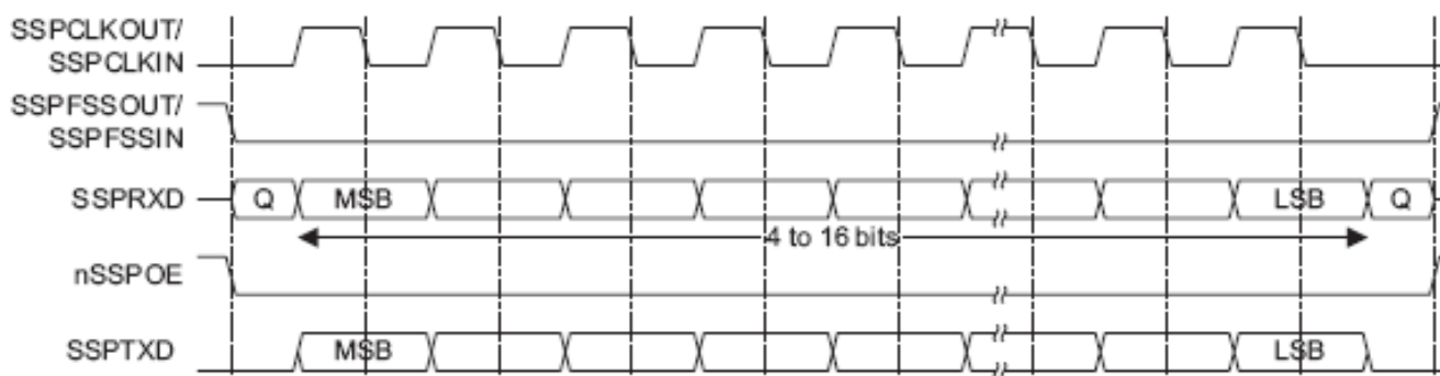
Рисунок 111 – Формат синхронного обмена протокола SPI, SPO=0, SPH=1
