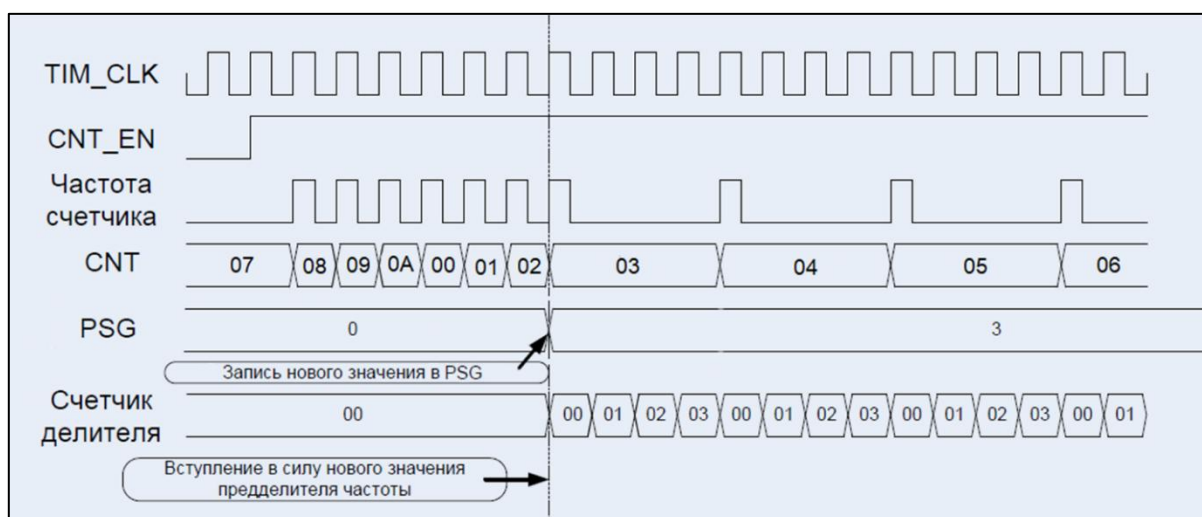
Рисунок 76 – Диаграмма работы счетчика: счет прямой (CNT_MODE[1:0] = 00, EVENT_SEL[3:0] = 0000, DIR = 0)
