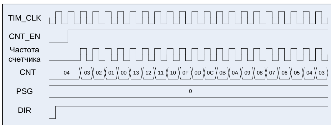
Рисунок 70 – Диаграммы работы таймера, счет обратный от 0x13 до 0, стартовое значение 0x04
