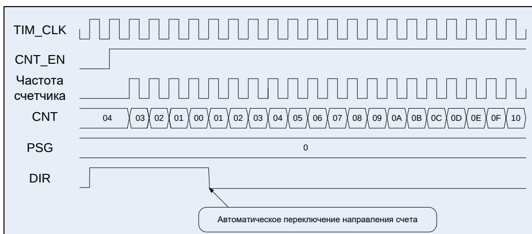
Рисунок 72 – Диаграммы работы таймера, счет двунаправленный, сначала обратный
