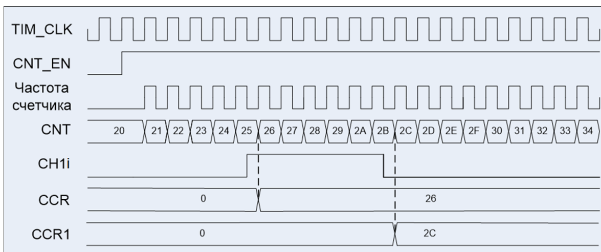
Рисунок 85 – Диаграмма захвата события со входа канала 1
