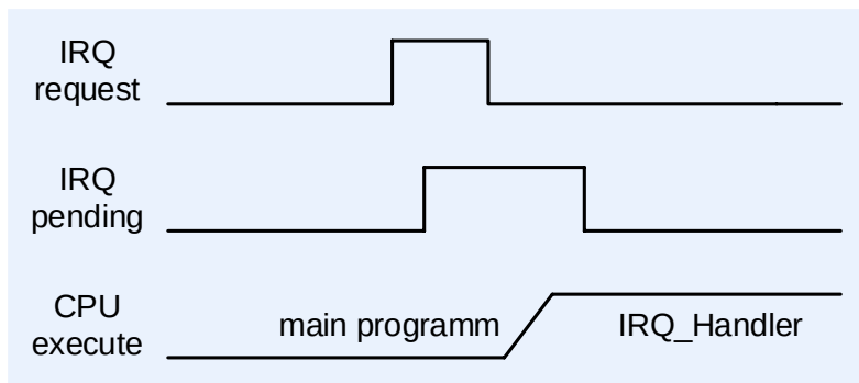
Рисунок 143 – Выставление отложенного запроса на прерывание и последующая его обработка
