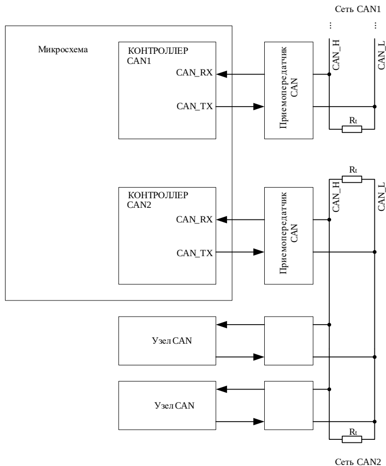
Рисунок 50 – Структурная блок – схема организации сети CAN
