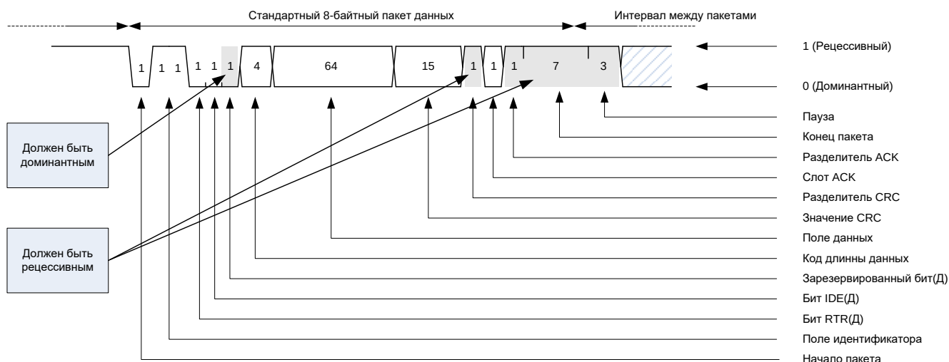
Рисунок 61 – Контроль формата пакета
