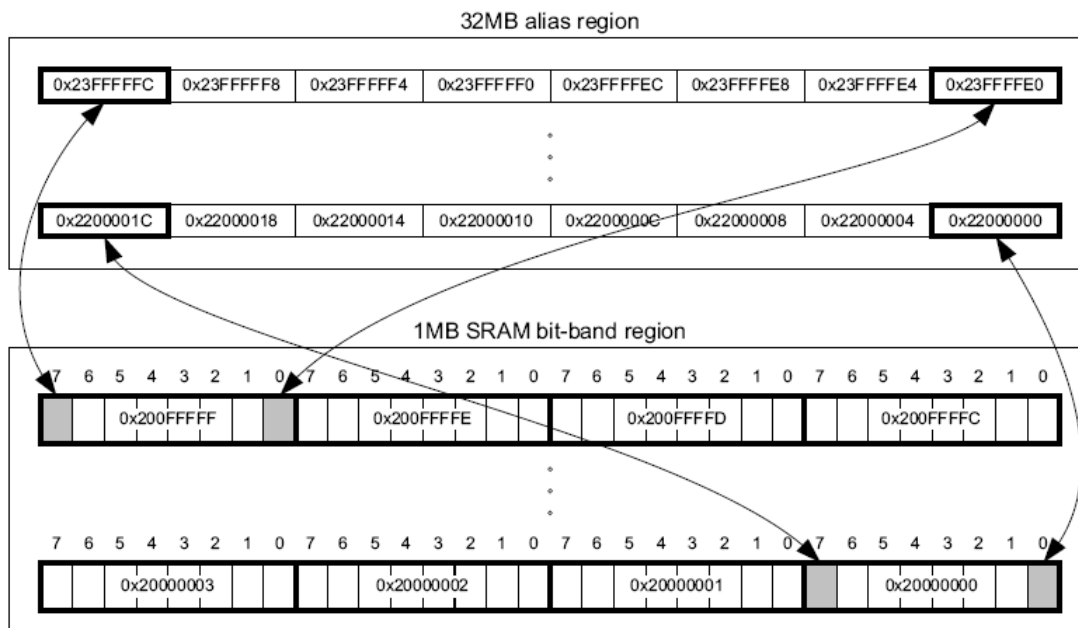
Рисунок 17 – Схема отображения региона bit-band alias в регионе bit-band region
