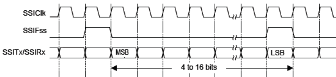
Рисунок 108 – Формат синхронного обмена протокола SSI (непрерывный обмен)
