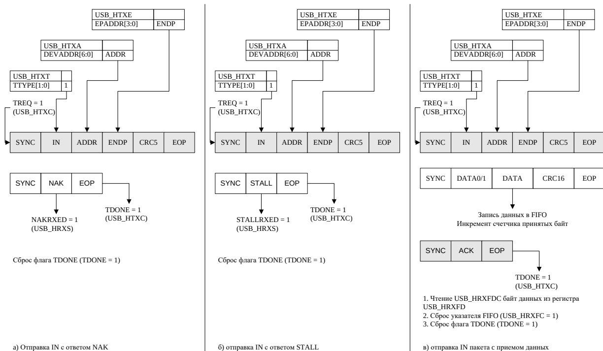
Рисунок 49 (а, б, в) – Транзакция IN (USB Host)
