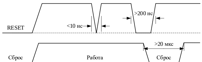
Рисунок 14 – Формирование сигнала сброса
