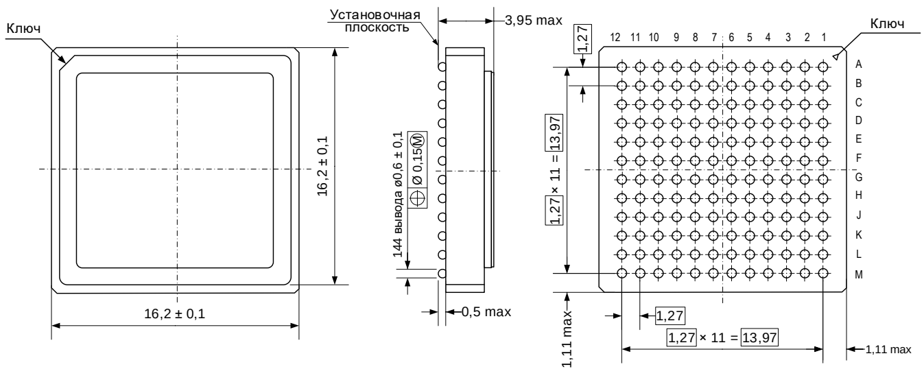
Рисунок 164 – Корпус МК 8307.144-АНЗ
