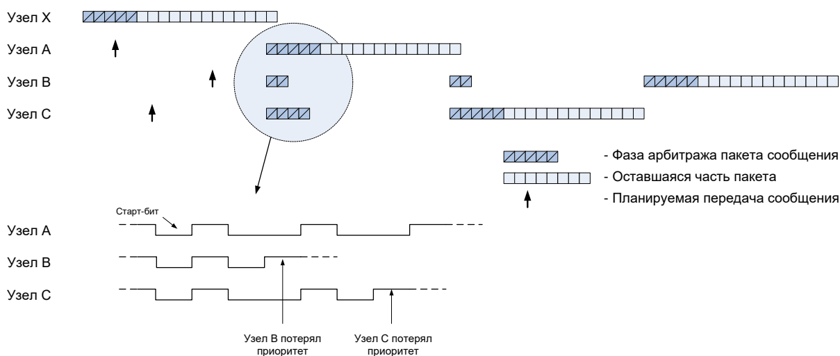
Рисунок 58 – Арбитраж на шине CAN
