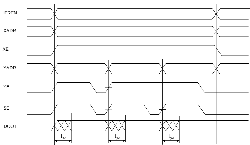
Рисунок 24 – Временная диаграмма чтения памяти
