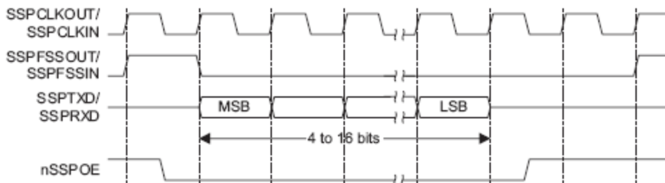
Рисунок 107 – Формат синхронного обмена протокола SSI (единичный обмен)
