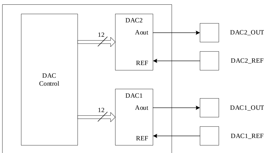
Рисунок 99 – Структурная схема контроллера ЦАП
