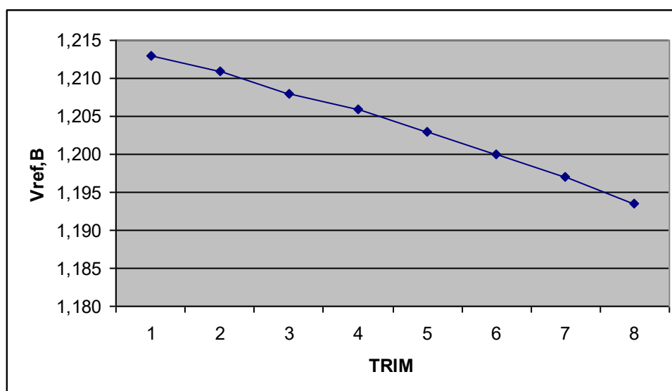
Рисунок 98 – Зависимость источника опорного напряжения от подстройки
