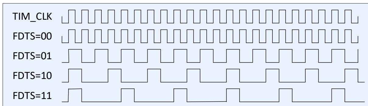
Рисунок 74 – Диаграмма тактовой частоты F_{DTS} в зависимости от значения FDTs[1:0] в регистре CNTRL
