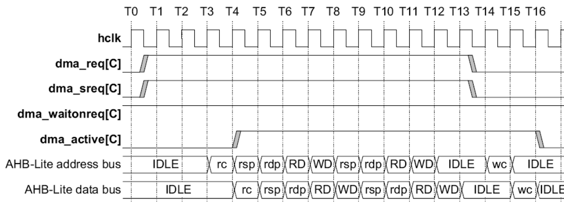
Рисунок 133 – Диаграмма работы контроллера DMA при использовании dma_waitonreq
