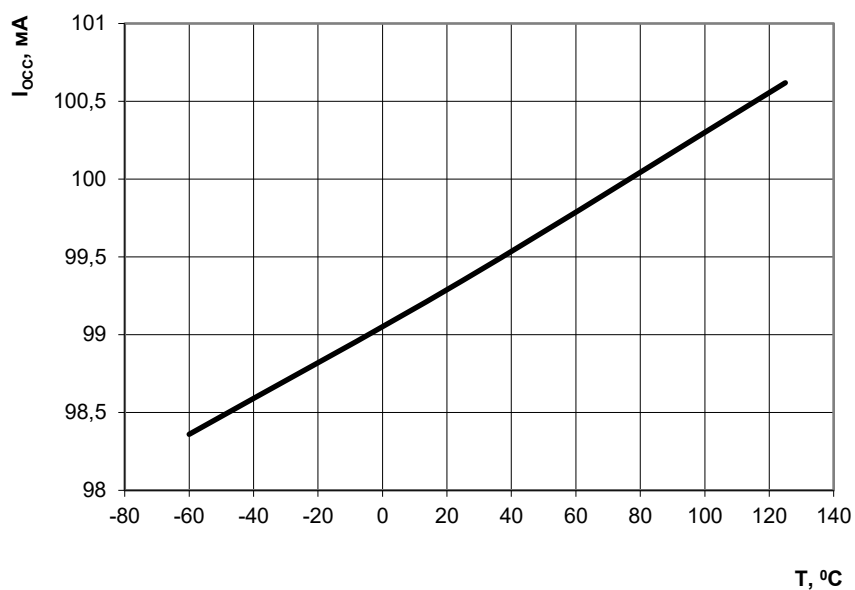
Рисунок 150 – Зависимость динамического тока потребления от температуры при: f_c = 80 МГц
