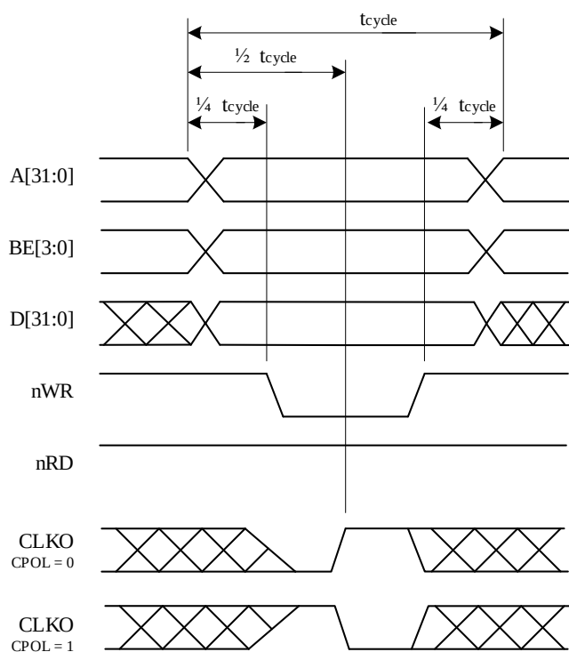
Рисунок 39 – Диаграмма записи
