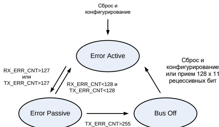
Рисунок 66 – Счетчики ошибок
