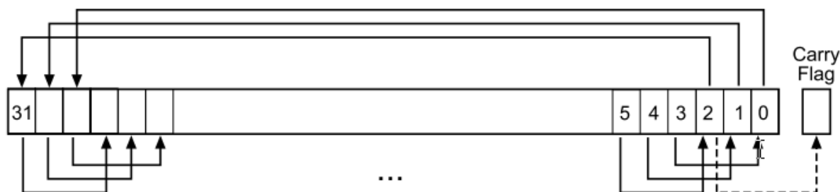
Рисунок 30 – Инструкция ROR # 3
