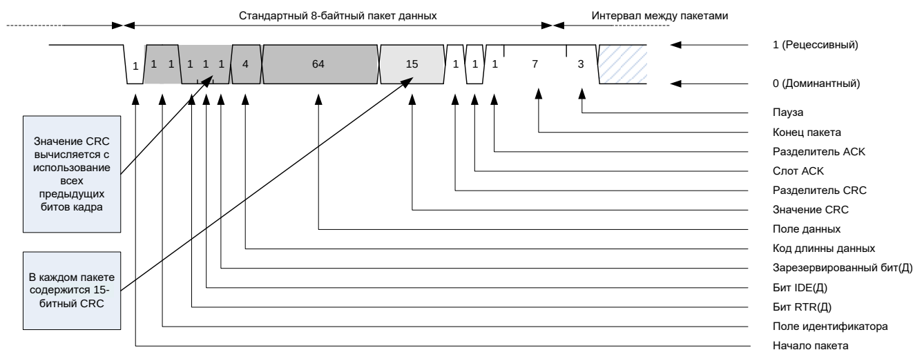
Рисунок 63 – Контроль CRC
