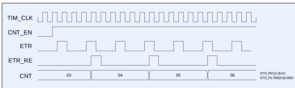
Рисунок 83 – Диаграмма тактирования со входа ETR, EVENT_SEL[3:0] = 1000
