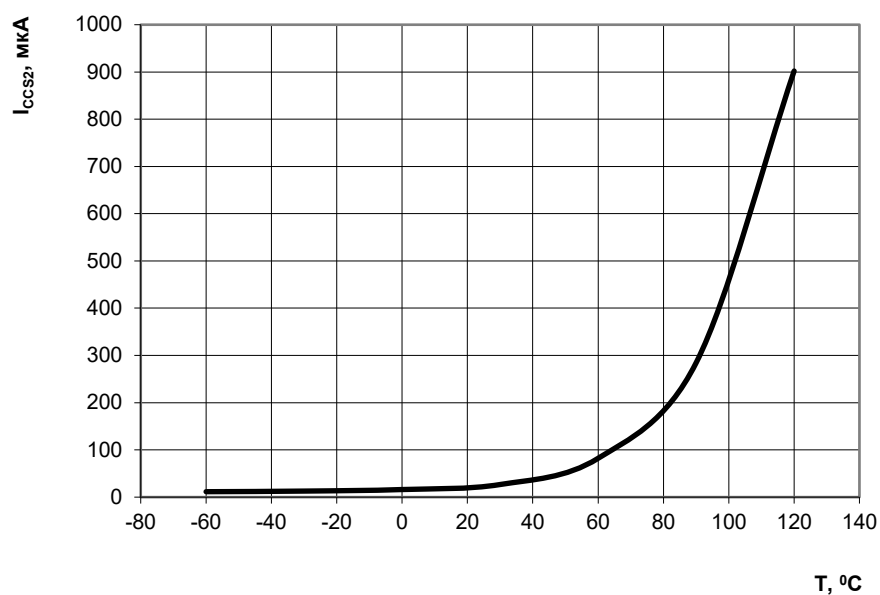
Рисунок 154 – Зависимость статического тока потребления в режиме покоя (регулятор напряжения включен) от температуры
