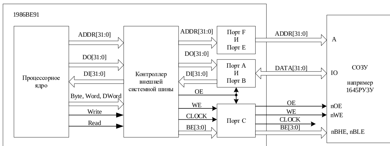
Рисунок 38 – Обмен по внешней системной шине
