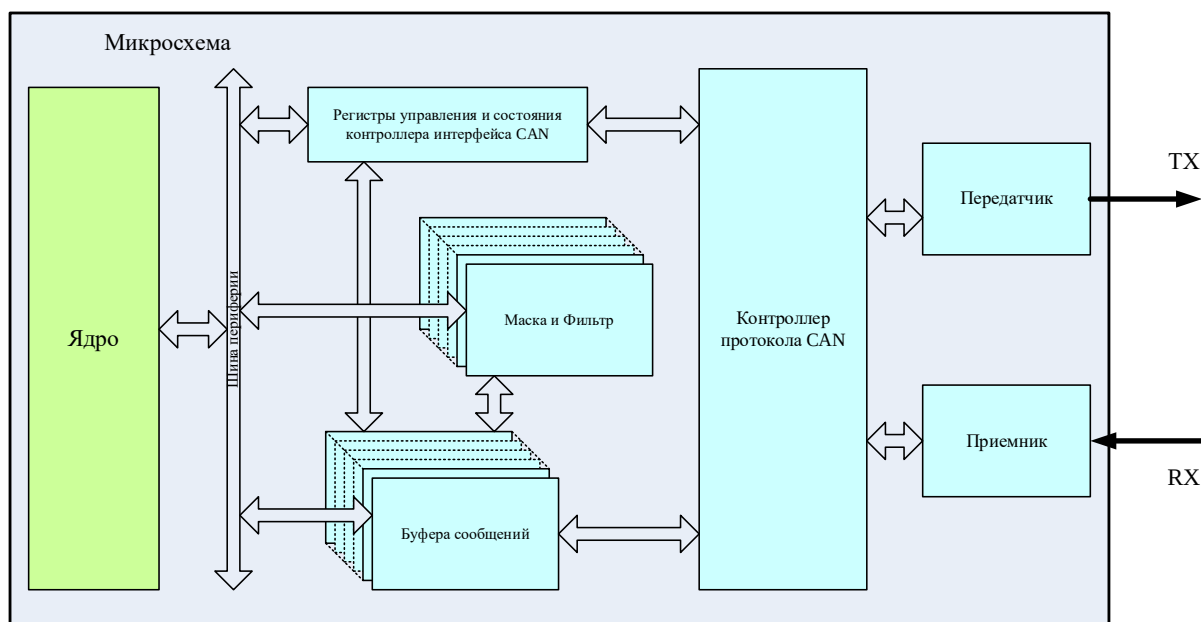
Рисунок 59 – Структурная блок-схема контроллера CAN
