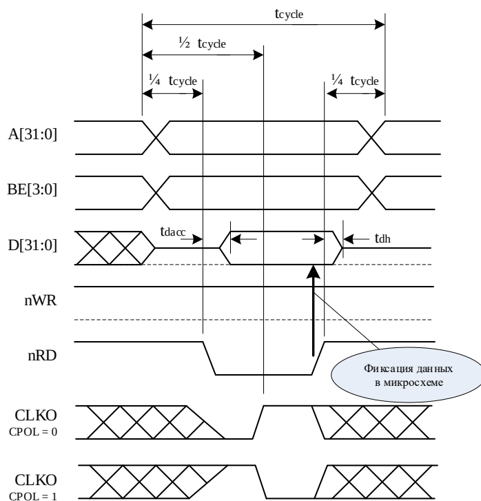
Рисунок 40 – Диаграмма чтения
