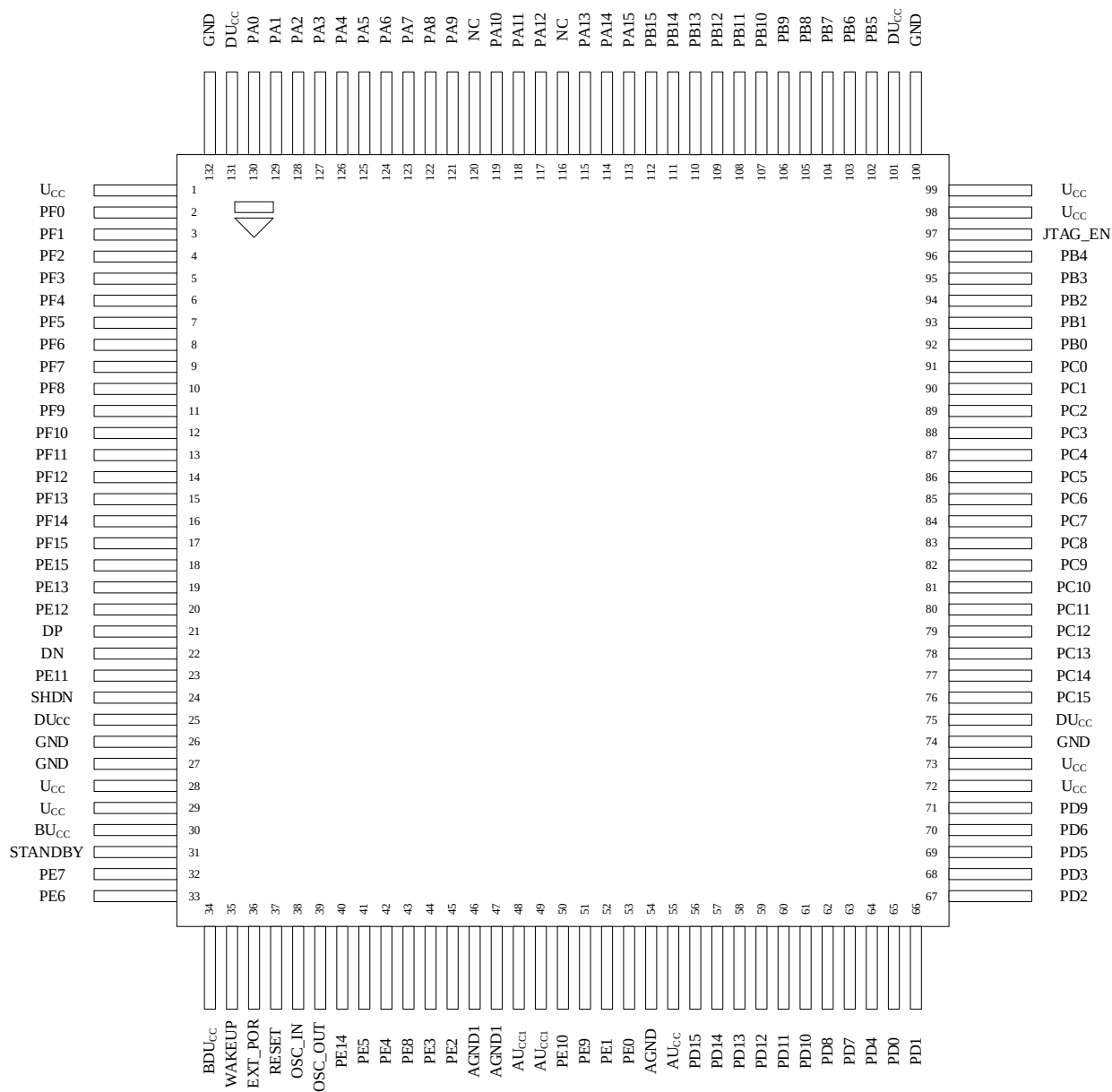
Рисунок 8 – Расположение выводов в 132-выводном корпусе 4229.132-3
